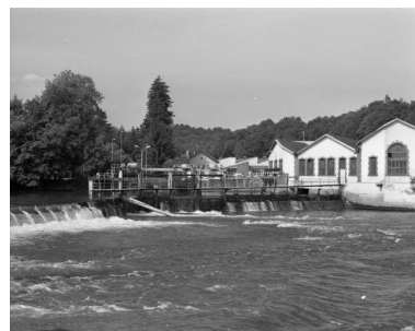
Entrepôt industriel (ancienne fonderie) et vannes du barrage depuis la rive droite. Phot. Jérôme Mongreville IVR43_20022500408X
