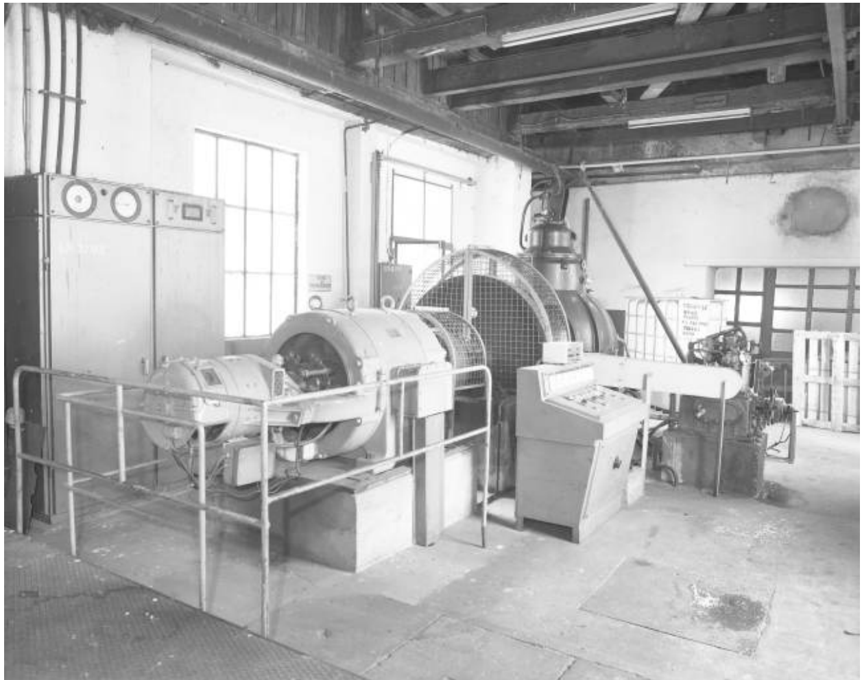
Turbine. Vue générale.
