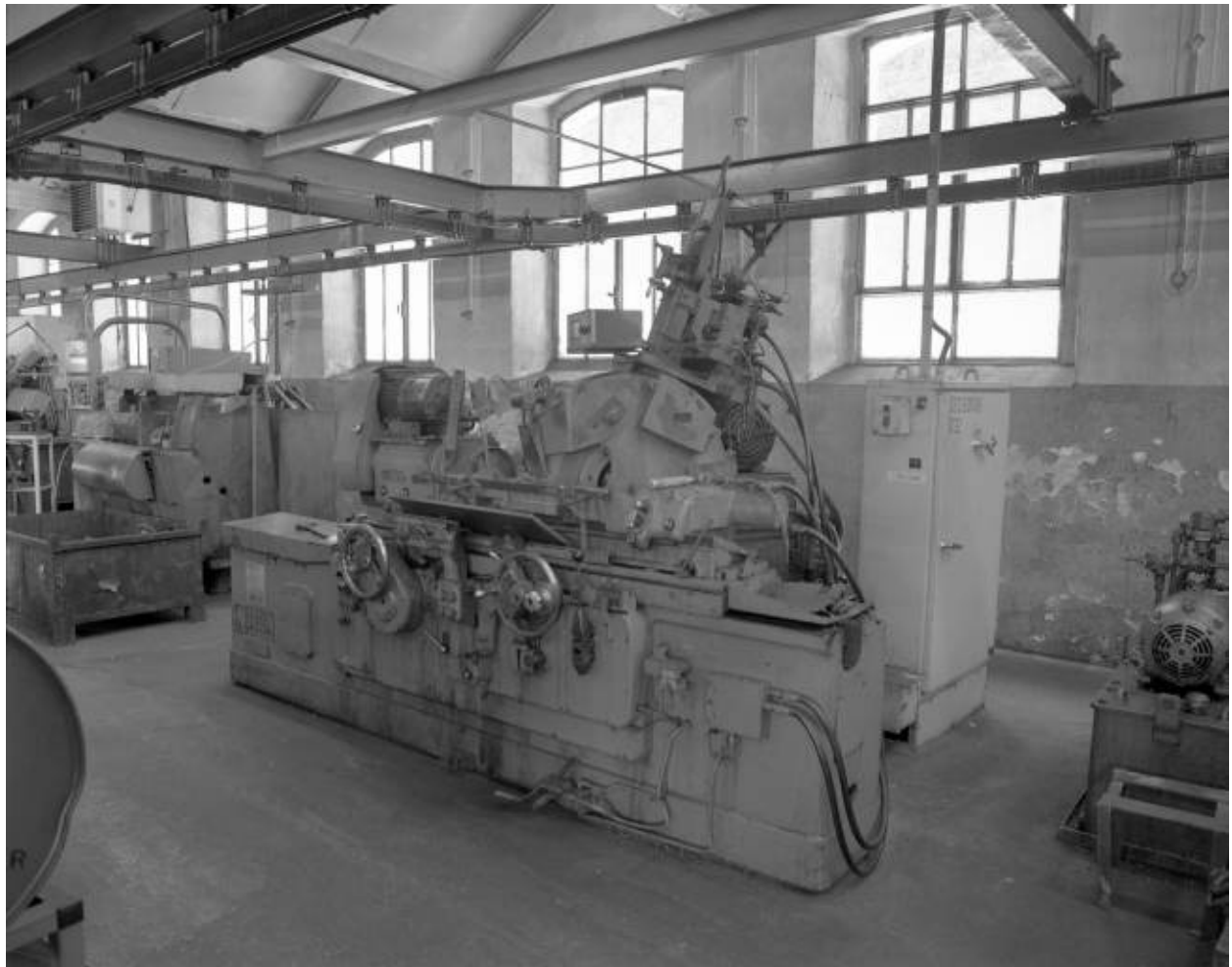
Rectifieuse Norton (atelier des fins de séries).
