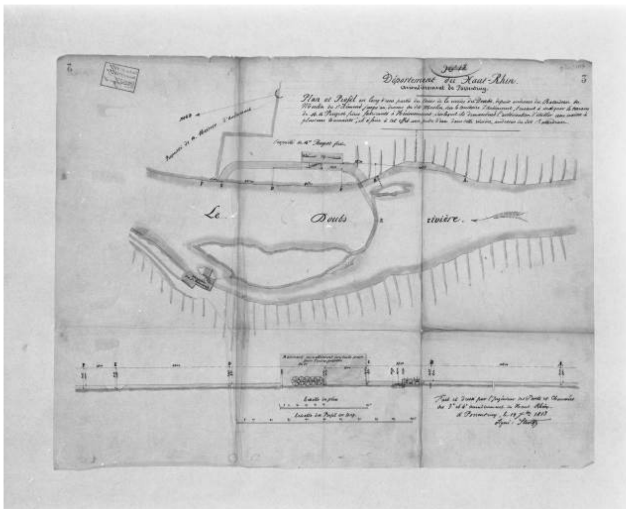
Plan et profil en long d'une partie du cours de la rivière du Doubs [...]. Dessin (plume, lavis), par Stroltz, le 19 décembre 1813, échelle 1:1000.
