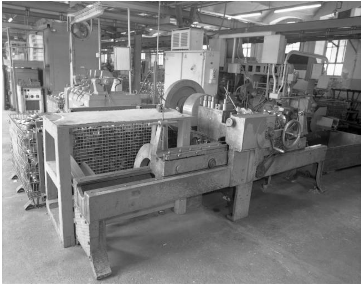
Redresseuse (atelier des fins de séries).
