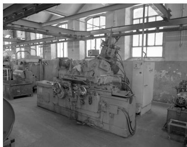
Rectifieuse Norton (atelier des fins de séries). Phot. Jérôme Mongreville IVR43_20022500420X
