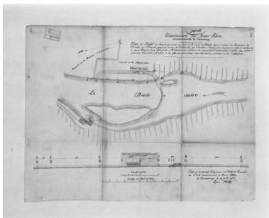
Plan et profil en long d'une partie du cours de la rivière du Doubs [...]. Dessin (plume, lavis), par Stoltz, le 19 décembre 1813, échelle 1:1000. Phot. Yves Sancey, Autr. Stoltz IVR43_20022500422X
