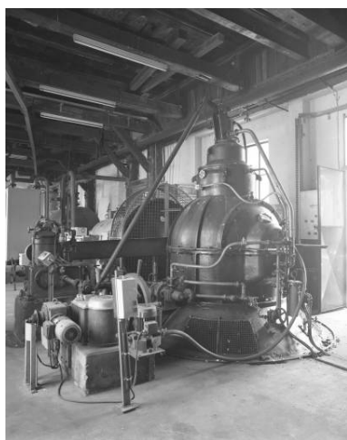
Turbine. Détail. Phot. Jérôme Mongreville IVR43_20022500380X
