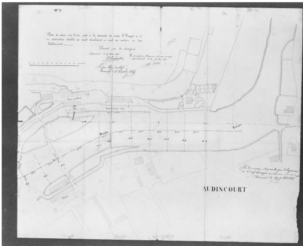
Plan des usines Sous Roche joint à la demande des sieurs Constant Peugeot et Cie [...]. Dessin (plume, lavis), signé Constant Peugeot et Cie, le 9 juin 1840, échelle 1:1250.
