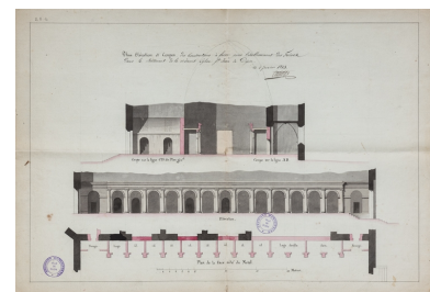
Plan des constructions à faire pour l'établissement des foires dans le bâtiment de la ci-devant église St Jean de Dijon [plan et élévation des aménagements intérieurs côté nord, et coupe transversale]. 4 janvier 1813. Phot. Pierre-Marie Barbe-Richaud, Autr. Caristie IVR26_2022100830NUC2A
