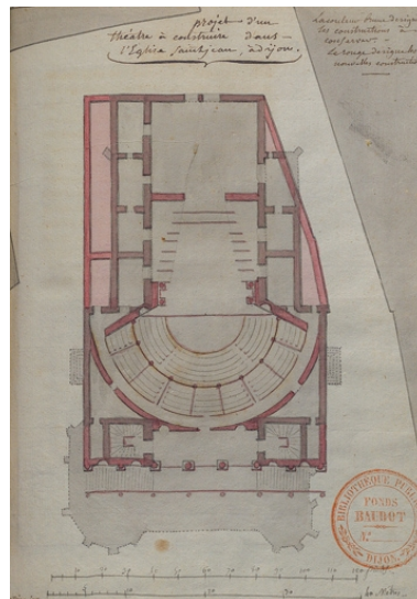
Projet d'un théâtre à construire dans l'église Saint-Jean, à Dijon [plan, d'après Pierre Joseph Antoine]. S.d. [décennie 1800]. Autr. Pierre Louis Baudot, Autr. Pierre Joseph Antoine IVR26_2022100859NUC2A
