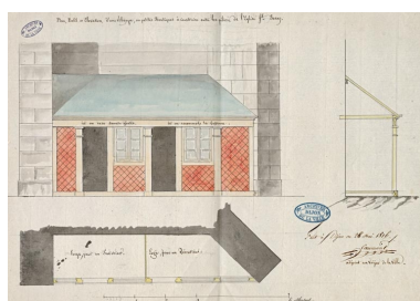
Plan, profil et élévation d'une échoppe, ou petites boutiques à construire entre les piliers de l'église St Jean. 28 mai 1816. Autr. Jacques Caumont IVR26_2022100761NUC4A
