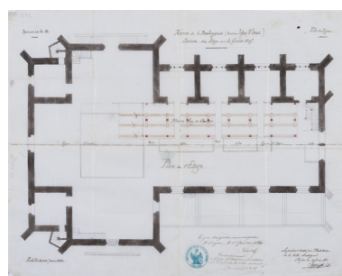
Réserve de la boulangerie (ancienne église St Jean). Création d'un étage sur la grande nef [plan]. 10 juin 1860. Phot. Pierre-Marie Barbe-Richaud, Autr. Jean Alphée Cyprien Scheffer IVR26_2022100832NUC2A
