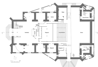
Plan du rez-de-chaussée. D'après un plan du 30 août 2013 fourni par le service des Données patrimoniales, direction Bâtiments et Energies de Dijon Métropole. Dess. Aline Thomas IVR26_20222100684NUDA
