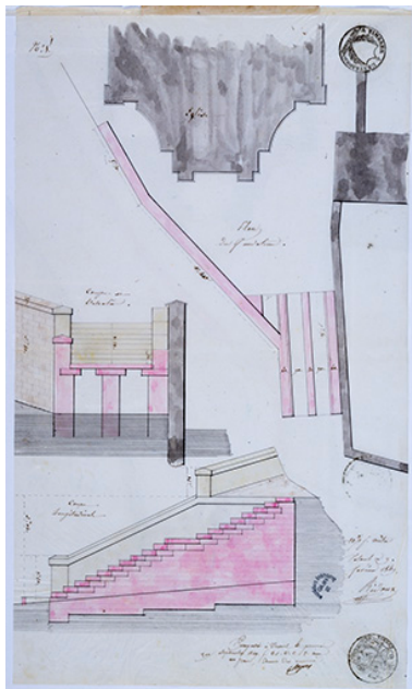
escalier du parvis de l'église Phot. Jérôme Mongreville, Autr. Jean-Baptiste Ridoux IVR43_20167001581NUC4A
