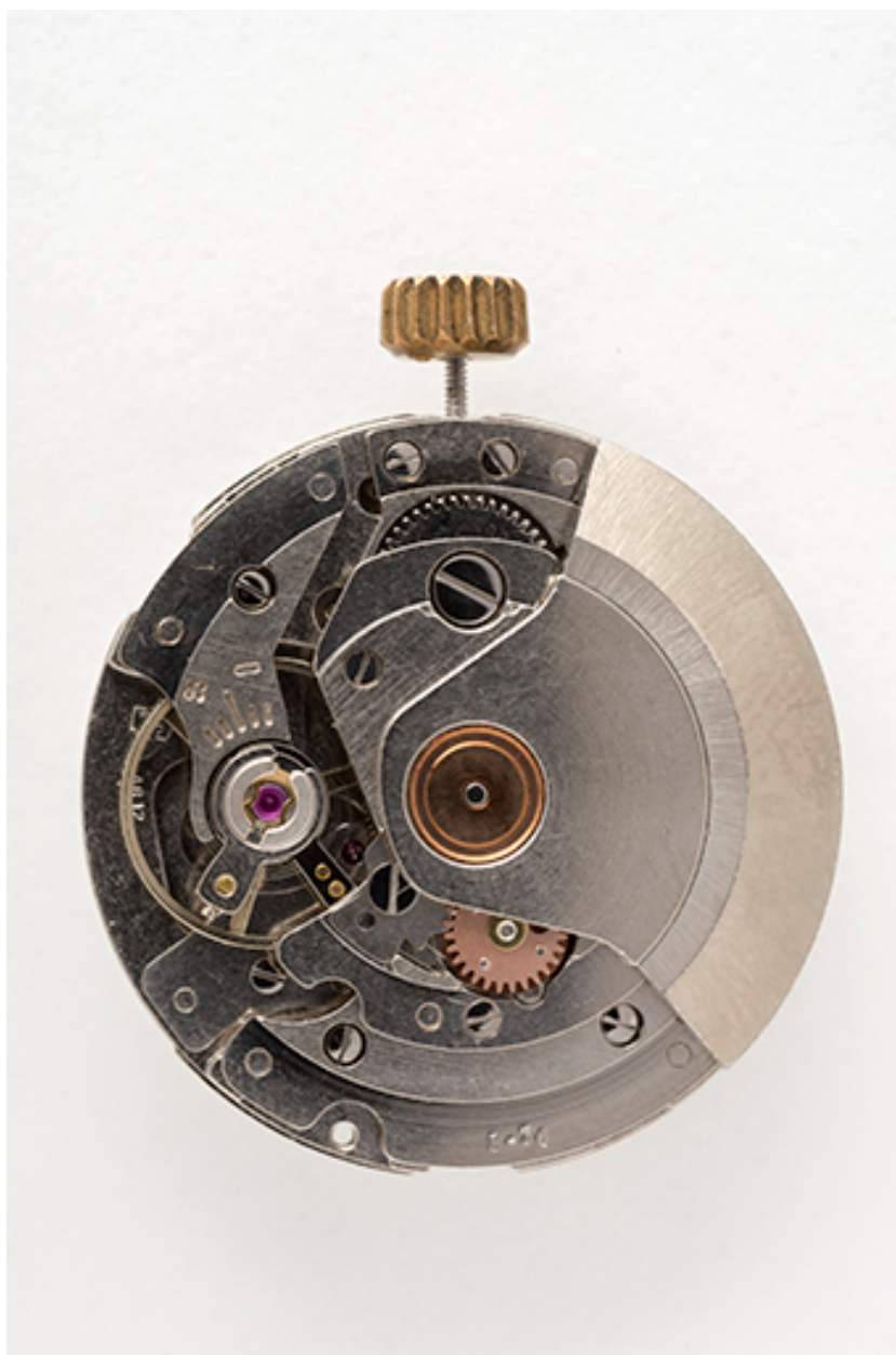
Mouvement FE 4612, vu côté ponts.
