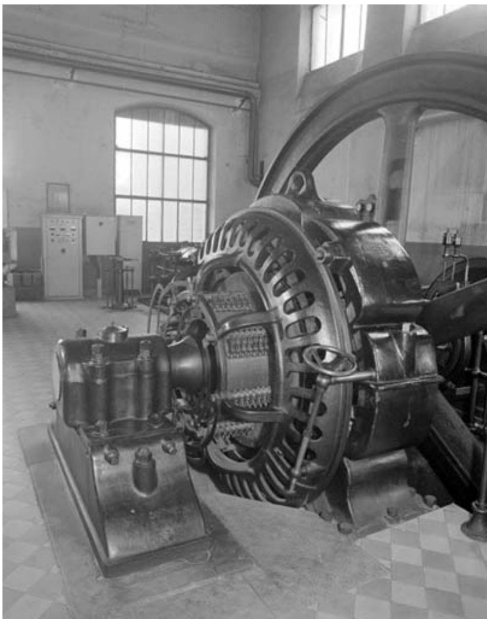
Salle des machines (10) : dynamo Schneider et Cie.
