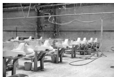
Atelier de coulage C (9) : bancs de coulage. Phot. Laurent Poupard IVR43_19893901134Z
