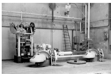
Atelier de préparation de la pâte (9) : pompes à barbotine. Agitateurs à barbotine au 1er plan ; pompe ancien modèle à gauche, pompes nouveau modèle au centre. Phot. Laurent Poupard IVR43_19893901132Z
