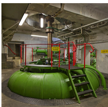
Centrale de Liebwillers : turbine du groupe n° 4.
