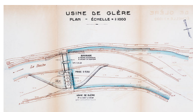
Aménagement du Doubs entre la frontière Suisse et Vaufrey [...] Usine de Glère. Plan général, 1er septembre 1922. Phot. Jérôme Mongreville, Autr. Compagnie générale d'Électricité IVR43_20132500568NUC4A
