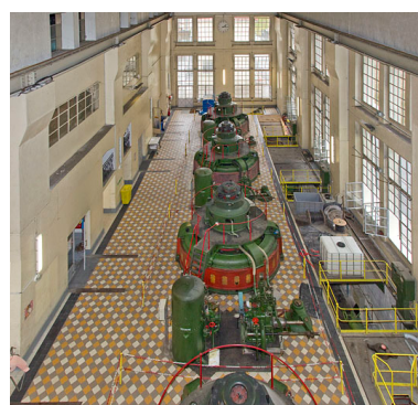
Centrale de Liebwillers : intérieur de la salle des machines.
