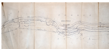
Projet d'aménagement hydro-électrique du Doubs entre le Saut-du-Doubs et le Moulin Delachaux. Chute du Châtelot.
