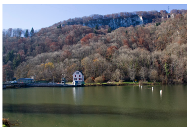
Barrage de Grosbois (commune de Soulce-Cernay) : vue d'ensemble depuis la rive gauche, en amont.
