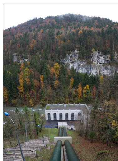
Centrale du Refrain (commune de Charquemont) : vue plongeante depuis le haut de la conduite forcée.
