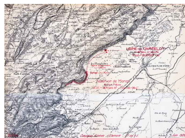
Projet d'aménagement hydro-électrique du Doubs entre le Saut-du-Doubs et le Moulin Delachaux. Chute du Châtelot. Carte d'État major, juin 1928. Phot. Jérôme Mongreville, Autr. Compagnie générale d'Électricité IVR43_20132500592NUC4A
