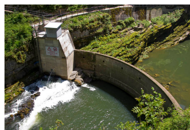
Barrage du Châtelot : barrage aval du bassin d'amortissement. Phot. Yves Sancey IVR43_20130000019NUC2A
