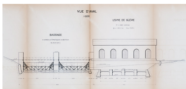
Aménagement du Doubs entre la frontière Suisse et Vaufrey [...] Usine de Glère. Vue d'aval, 1er septembre 1922. Phot. Jérôme Mongreville, Autr. Compagnie générale d'Électricité IVR43_20132500569NUC4A
