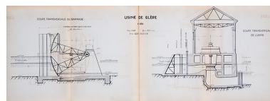
Aménagement du Doubs entre la frontière Suisse et Vaufrey [...] Usine de Glère. Coupes des principaux ouvrages, 1er septembre 1922. Phot. Jérôme Mongreville, Autr. Compagnie générale d'Électricité IVR43_20132500563NUC4A
