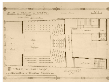
Ville de Louhans. Restauration du théâtre municipal. Plan au niveau des balcons. 20 octobre 1930. Phot. Pierre-Marie Barbe-Richaud, Autr. Georges Lamirand IVR26_20267100272NUC4A
