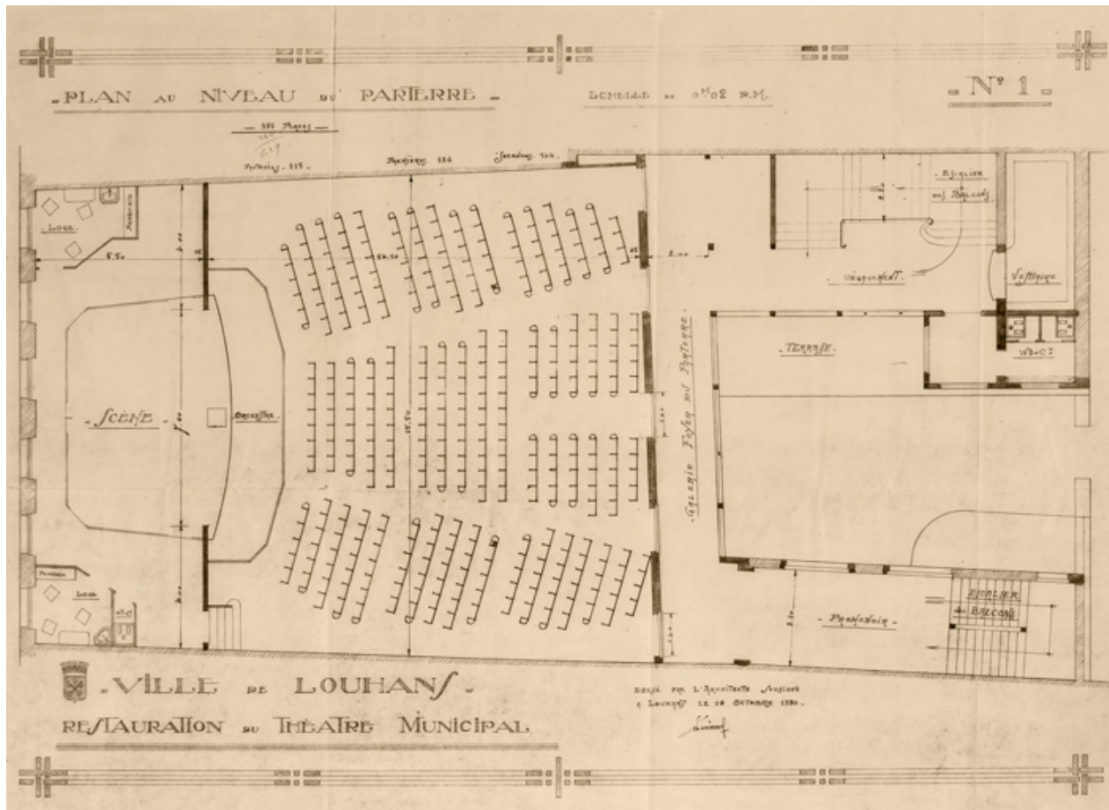
Ville de Louhans. Restauration du théâtre municipal. Plan au niveau du parterre. 10 octobre 1930.
