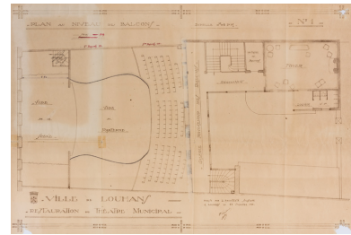
Ville de Louhans. Restauration du théâtre municipal. Plan au niveau des balcons. 28 janvier 1929, rectifié le 25 octobre 1930. Phot. Pierre-Marie Barbe-Richaud, Autr. Georges Lamirand IVR26_20267100275NUC4A
