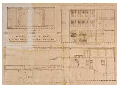
Ville de Louhans. Restauration du théâtre municipal. Coupes. 30 janvier 1930. Phot. Pierre-Marie Barbe-Richaud, Autr. Georges Lamirand IVR26_20267100278NUC4A
