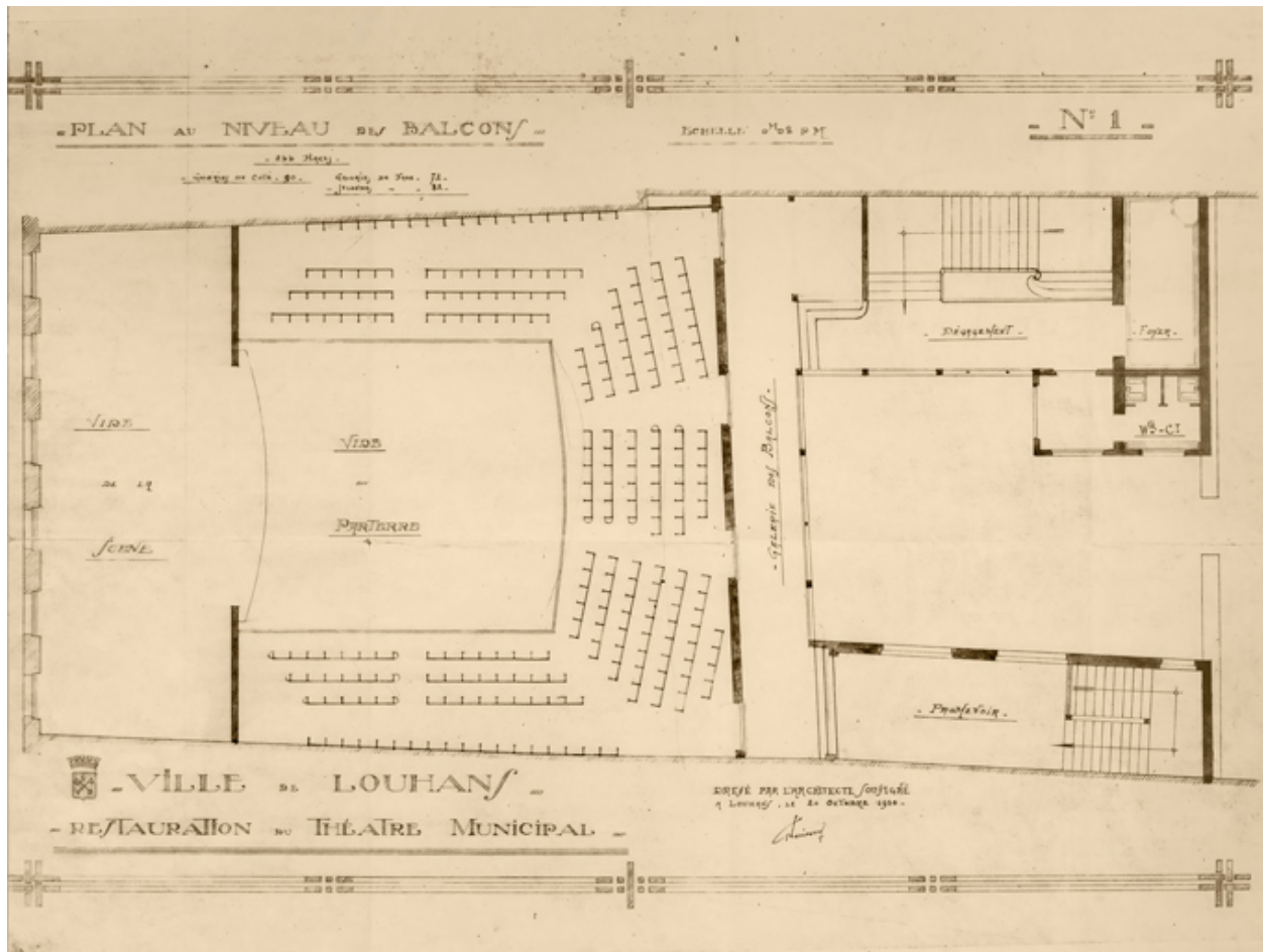
Ville de Louhans. Restauration du théâtre municipal. Plan au niveau des balcons. 20 octobre 1930.
