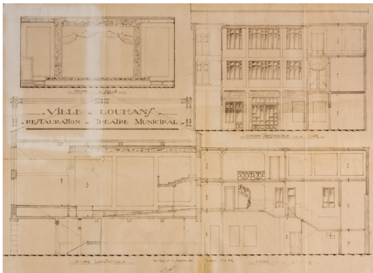
Ville de Louhans. Restauration du théâtre municipal. Coupes. 30 janvier 1930.
