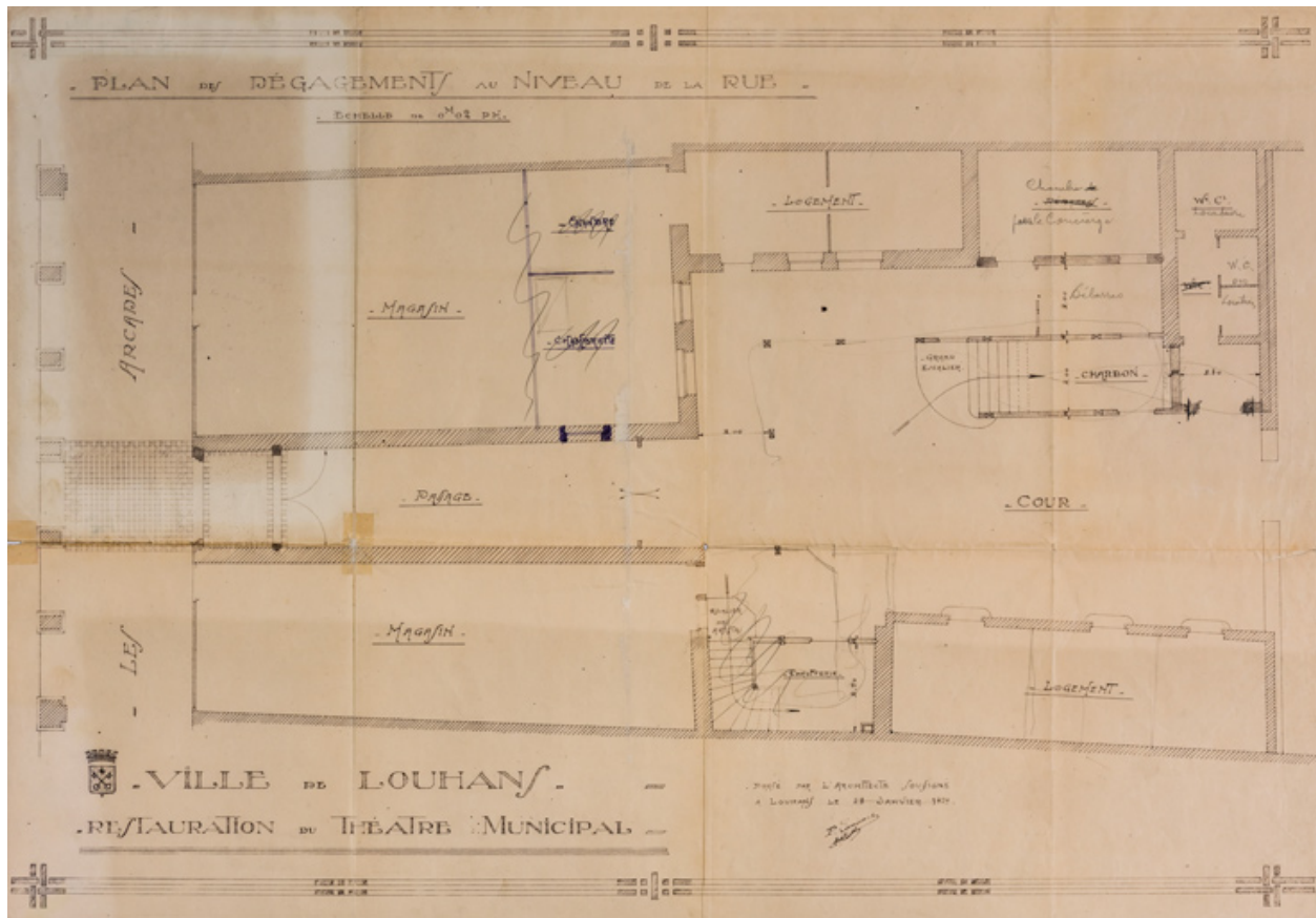
Ville de Louhans. Restauration du théâtre municipal. Plan des dégagements au niveau de la rue. 28 janvier 1929, rectifié le 25 octobre 1930.
