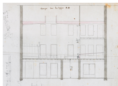
Projet des ouvrages supplémentaires à faire pour achever les batimens, sur la rue, de l'ancien collège de la ville de Louhans. Coupe sur la ligne AB. 2 octobre 1854. Phot. Pierre-Marie Barbe-Richaud, Autr. Gaguin IVR26_20267100284NUC4A
