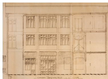
Ville de Louhans. Restauration du théâtre municipal. Coupes [détail]. Coupe transversale sur la cour. 30 janvier 1930. Phot. Pierre-Marie Barbe-Richaud, Autr. Georges Lamirand IVR26_20267100280NUC4A
