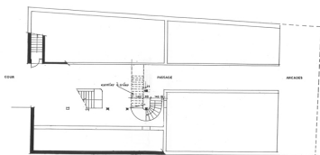
PLAN NIVEAU -1 Etat actuel éch. 1 cm / p.m.
