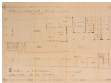
Ville de Louhans. Restauration du théâtre municipal. Plan des dégagements. 10 octobre 1930. Phot. Pierre-Marie Barbe-Richaud, Autr. Georges Lamirand IVR26_20267100276NUC4A
