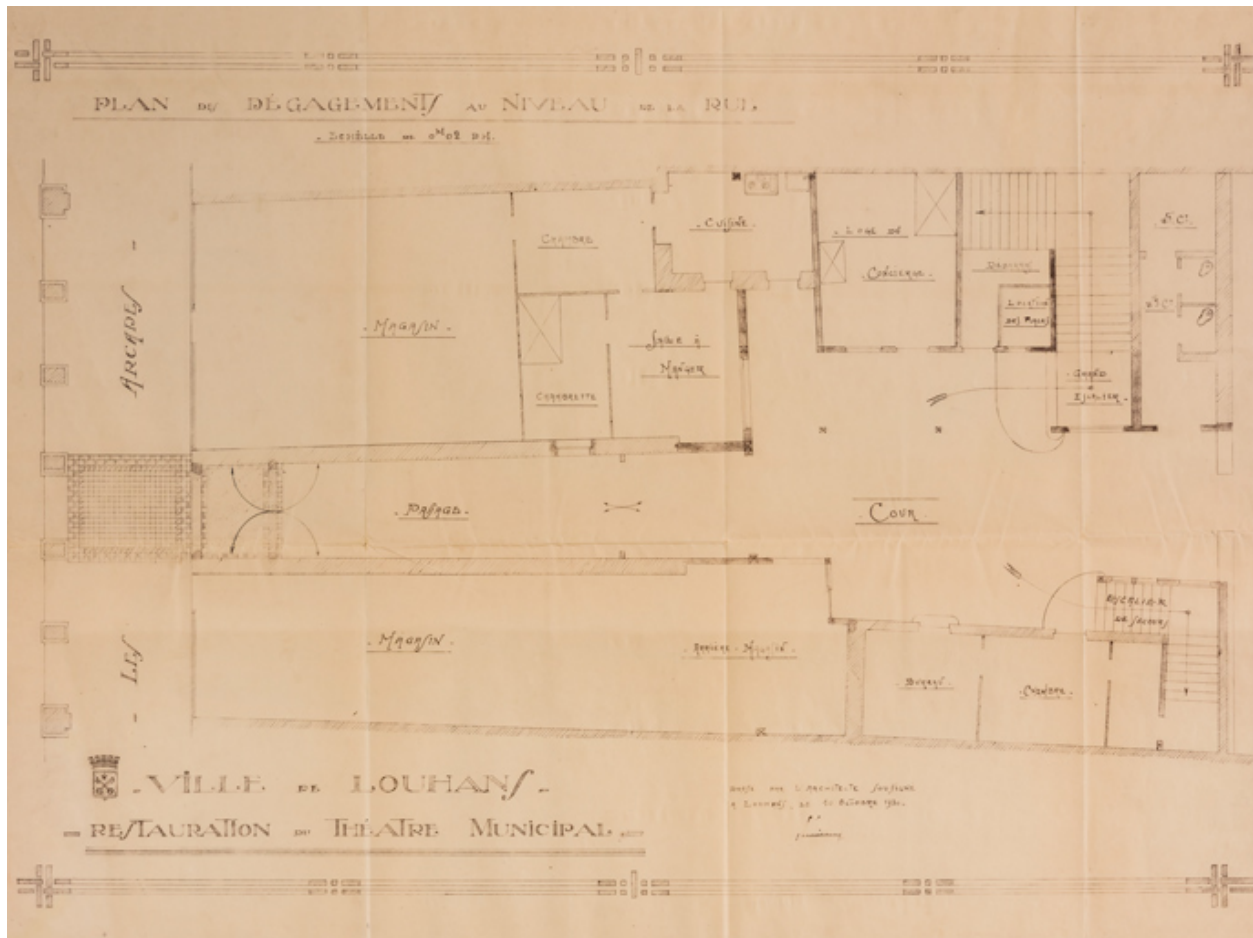
Ville de Louhans. Restauration du théâtre municipal. Plan des dégagements. 10 octobre 1930.
