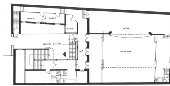
PLAN NIVEAU 0 Etat actuel éch. 1 cm / p.m.
