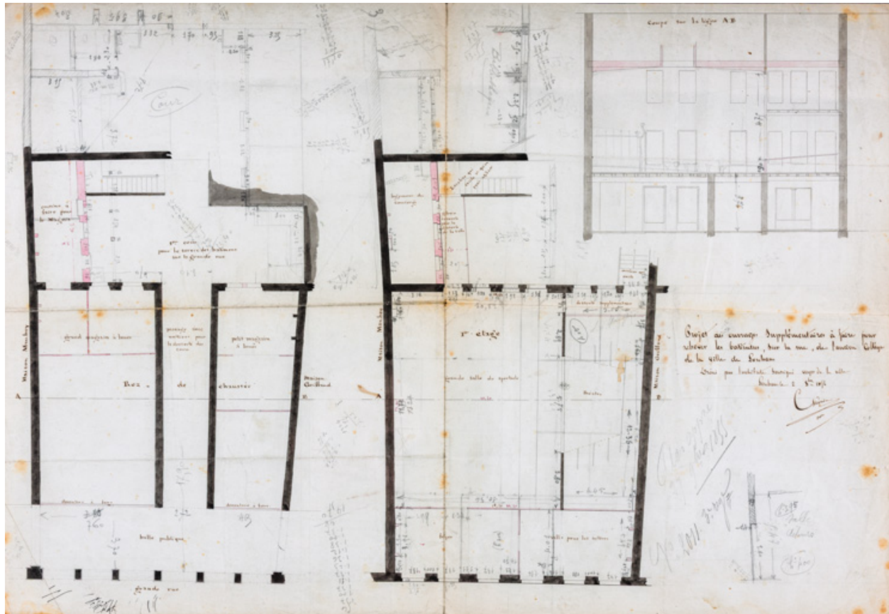
Projet des ouvrages supplémentaires à faire pour achever les batimens, sur la rue, de l'ancien collège de la ville de Louhans. 2 octobre 1854.
