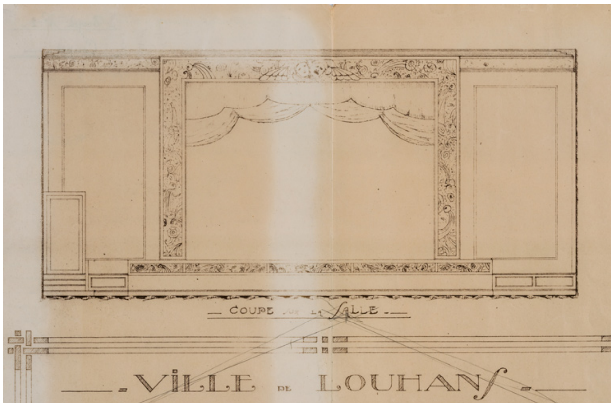
Ville de Louhans. Restauration du théâtre municipal. Coupes [détail]. Coupe sur la salle. 30 janvier 1930.
