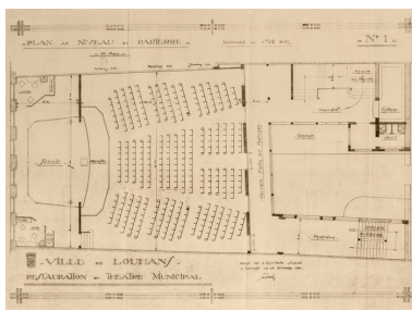
Ville de Louhans. Restauration du théâtre municipal. Plan au niveau du parterre. 10 octobre 1930. Phot. Pierre-Marie Barbe-Richaud, Autr. Georges Lamirand IVR26_20267100273NUC4A
