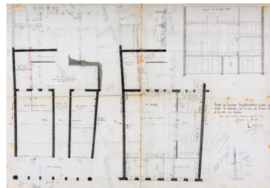
Projet des ouvrages supplémentaires à faire pour achever les bâtiments, sur la rue, de l'ancien collège de la ville de Louhans. 2 octobre 1854. Phot. Pierre-Marie Barbe- Richaud, Autr. Gaguin IVR26_20267100281NUC4A
