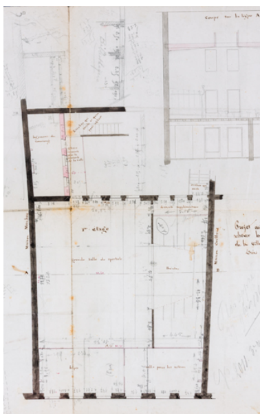
Projet des ouvrages supplémentaires à faire pour achever les batimens, sur la rue, de l'ancien collège de la ville de Louhans. 1er étage. 2 octobre 1854. Phot. Pierre-Marie Barbe-Richaud, Autr. Gaguin IVR26_20267100283NUC4A
