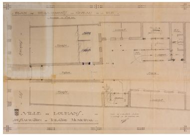
Ville de Louhans. Restauration du théâtre municipal. Plan des dégagements au niveau de la rue. 28 janvier 1929, rectifié le 25 octobre 1930. Phot. Pierre-Marie Barbe-Richaud, Autr. Georges Lamirand IVR26_20267100277NUC4A
