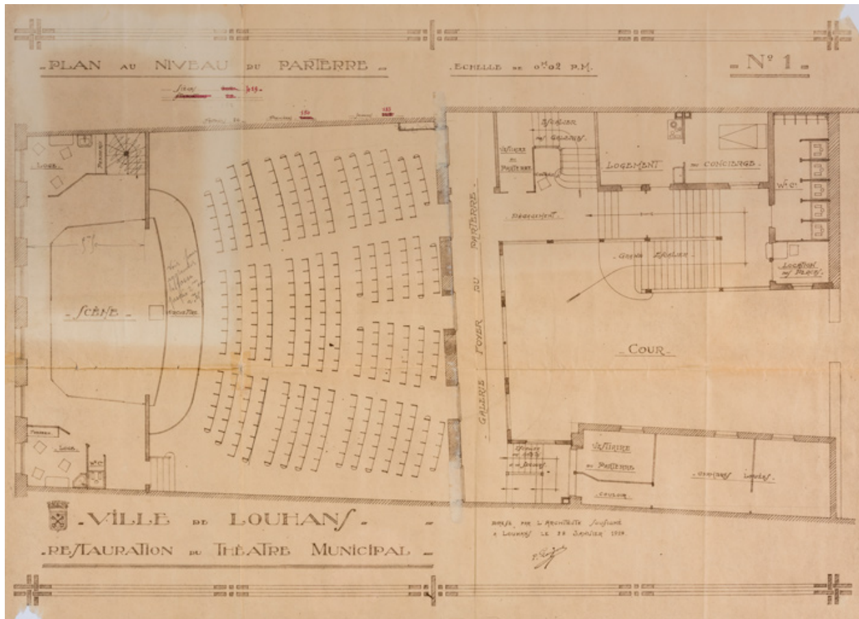
Ville de Louhans. Restauration du théâtre municipal. Plan au niveau du parterre. 28 janvier 1929, rectifié le 25 octobre 1930.
