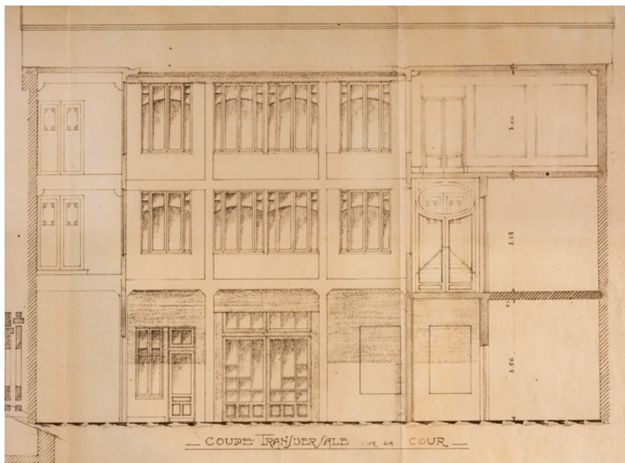
Ville de Louhans. Restauration du théâtre municipal. Coupes [détail]. Coupe transversale sur la cour. 30 janvier 1930.
