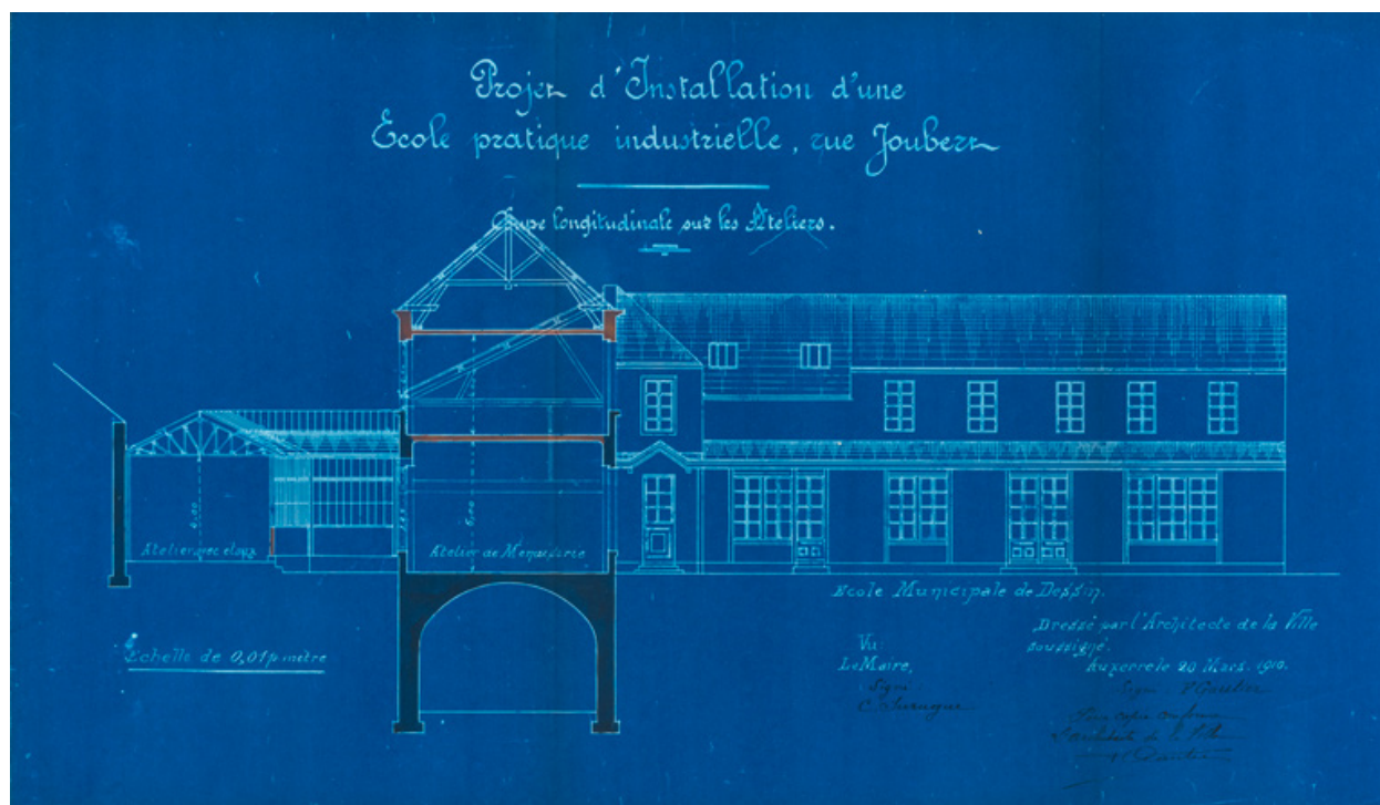
Ville d'Auxerre. Service des travaux et de la voirie. Ecole pratique d'industrie. Coupe longitudinale sur les ateliers. 20 mars 1910.
