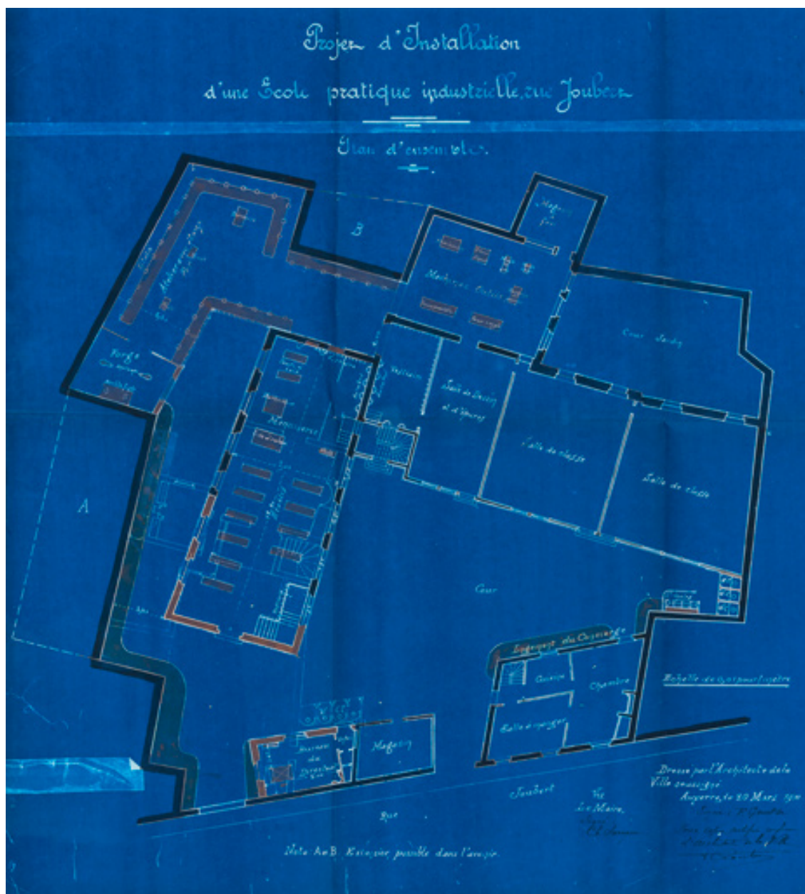
Ville d'Auxerre. Service des travaux et de la voirie. Ecole pratique d'industrie. Plan d'ensemble. 20 mars 1910.
