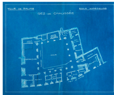
Projet d'aménagement de l'école Voltaire en école primaire supérieure. Plan du rez-de-chaussée, s.d. [1921].
