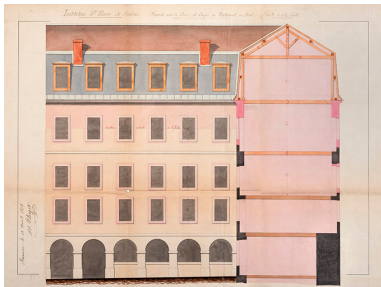
Institution Sainte-Marie de Salins. Façade sur la cour et coupe du bâtiment nord, 1879. Phot. Jérôme Mongreville, Autr. Alexandre Clerget IVR43_20233900902NUC4A
