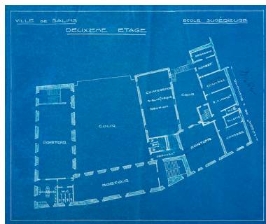
Projet d'aménagement de l'école Voltaire en école primaire supérieure. Plan du deuxième étage, s.d. [1921].
