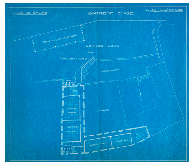
Projet d'aménagement de l'école Voltaire en école primaire supérieure. Plan du quatrième étage, s.d. [1921].
