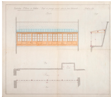
Institution Sainte-Marie de Salins. Projet de passage couvert entre les deux bâtiments, s.d. [1879]. Phot. Jérôme Mongreville IVR43_20233900903NUC4A
