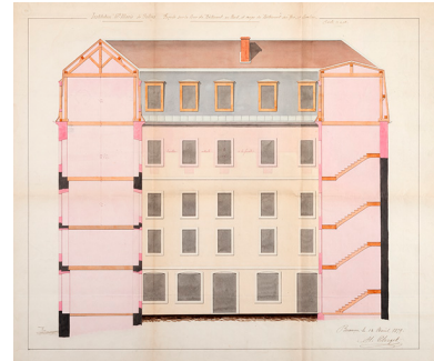
Institution Sainte-Marie de Salins. Façade sur la cour du bâtiment au nord, et coupe du bâtiment sur rue, 1879. Phot. Jérôme Mongreville, Autr. Alexandre Clerget IVR43_20233900901NUC4A
