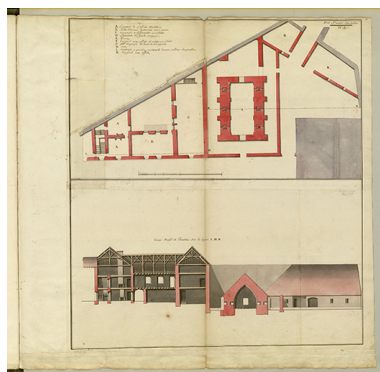
Fol. 15 Fort Saint-André-sur-Salins : plans, coupe, profil et élévation (magasin pour 60,000 milliers de poudre). 1756. IVR43_20243900503NUC4A
