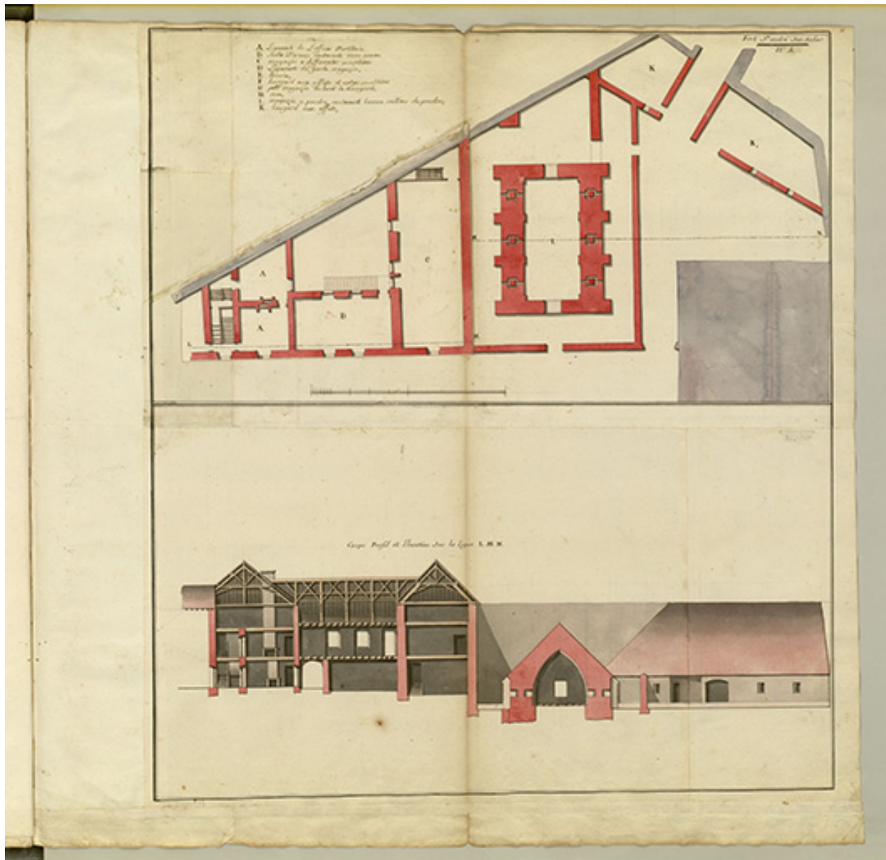
Fol. 15 Fort Saint-André-sur-Salins : plans, coupe, profil et élévation (magasin pour 60,000 milliers de poudre). 1756.
