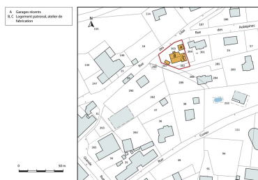
Plan-masse et de situation. Extrait du plan cadastral, 2015, section AC. Dess. Mathias Papigny IVR43_20152500653NUDA
