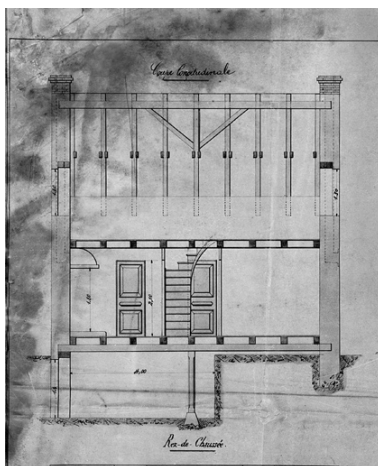
Habitation ouvrière. Cité Chatelot [coupe longitudinale]. Phot. Yves Sancey
