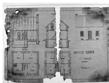
Habitation ouvrière. Cité Chatelot [plan, coupe, élévation]. Phot. Yves Sancey IVR43_19849000005X
