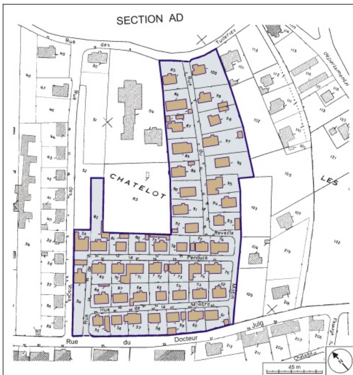
Plan-masse et de situation. Extrait du plan cadastral, 1979, section AI, 1:1500.
