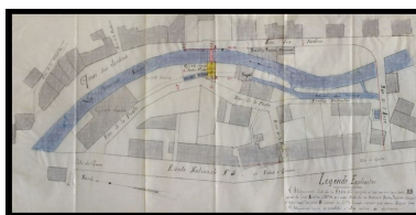
Etablissement d'une passerelle sur la Bienne pour faire communiquer la Rue des Jardins à la Rue de la Poste [...], 1893. Dessin sur calicot (plume, lavis), 30 janvier 1893, échelle 1:500. Phot. Yves Sancey, Autr. Emile (agent voyer) NEPASUTILISERJorez IVR43_20103900074NUC2A
