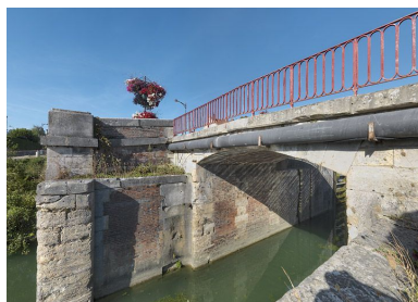
Le pont sur écluse : détail des maçonneries avec l'échelle de crues.
