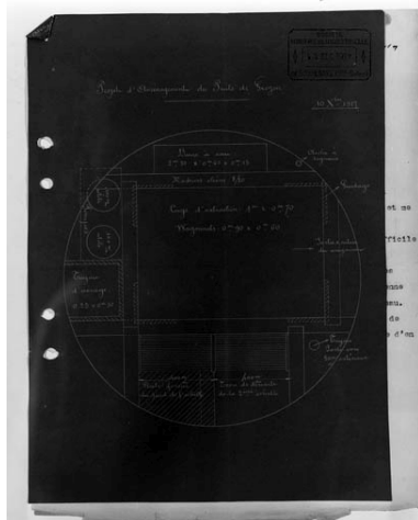
Projet d'aménagement du puits de Grozon. Phot. Jérôme Mongreville IVR43_19963901802V
