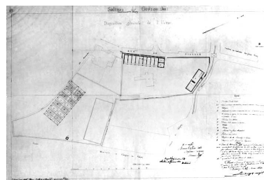
Salines de Grozon (Jura). Disposition générale de l'Usine. Phot. Jérôme Mongreville, Phot. Delize, Phot. Thomas, Phot. Boucard IVR43_19963901780V
