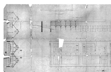
Projet de reconstruction du bâtiment et de l'atelier de formation de la saline de Grozon. Phot. Jérôme Mongreville, Autr. Gouget IVR43_19963901776V
