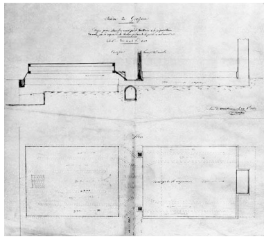
Saline de Grozon. Projet pour chauffer une poêle destinée à la préparation des eaux, par la vapeur et la chaleur perdue de la poêle à alimenter. Phot. Jérôme Mongreville, Autr. Gouget IVR43_19963901774V
