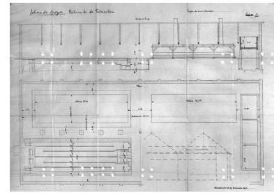
Saline de Grozon. Bâtiment de fabrication. Projet de reconstruction. Phot. Jérôme Mongreville IVR43_19963901770V
