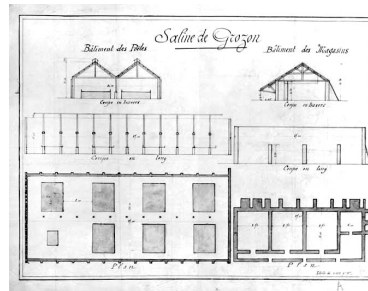
[Plan, coupe transversale et coupe longitudinale du bâtiment des poêles et du bâtiment des magasins]. Phot. Jérôme Mongreville IVR43_19963901775V
