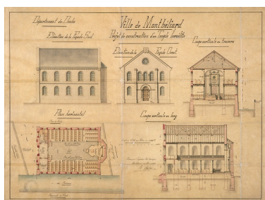
Projet de construction d'un temple israélite, 1888. Phot. Jérôme Mongreville, Autr. Charles-Frédéric (architecte) Surleau IVR43_19872500223XA
