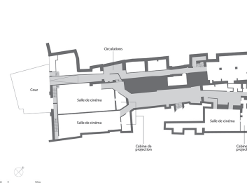
Plan au sous-sol. D'après un plan de la SMCI levé en décembre 2006 par François Gaume et complété en 2018 par le cabinet Coquard, 1/100 réduit à 1/250.
