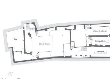
Plan au rez-de-chaussée. D'après un plan de la SMCI levé en décembre 2006 par François Gaume et complété en 2018 par le cabinet Coquard, 1/100 réduit à 1/250.
