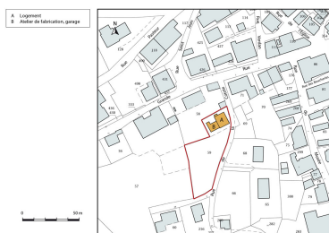
Plan-masse et de situation. Dess. Mathias Papigny IVR43_20162501518NUDA
