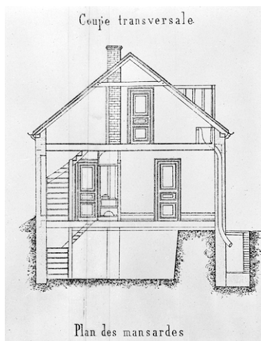
Maisons bâties à Beaucourt (Haut-Rhin) [...] : coupe transversale. Phot. Yves Sancey IVR43_19829000331V
