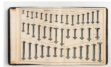
Boulons têtes rondes, carrées & à losanges [planche de catalogue], 1835. Phot. Sonia Dourlot IVR43_20209000024NUC4A
