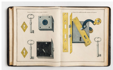
Serrures [... : planche de catalogue], 1835.
