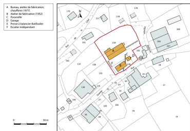
Plan-masse et de situation. Extrait du plan cadastral, 2013, section AC. Dess. Mathias Papigny IVR43_20142501531NUDA
