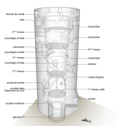
Le donjon vu en coupe. Dess. Mathias Papigny IVR43_20177001183NUDAQ
