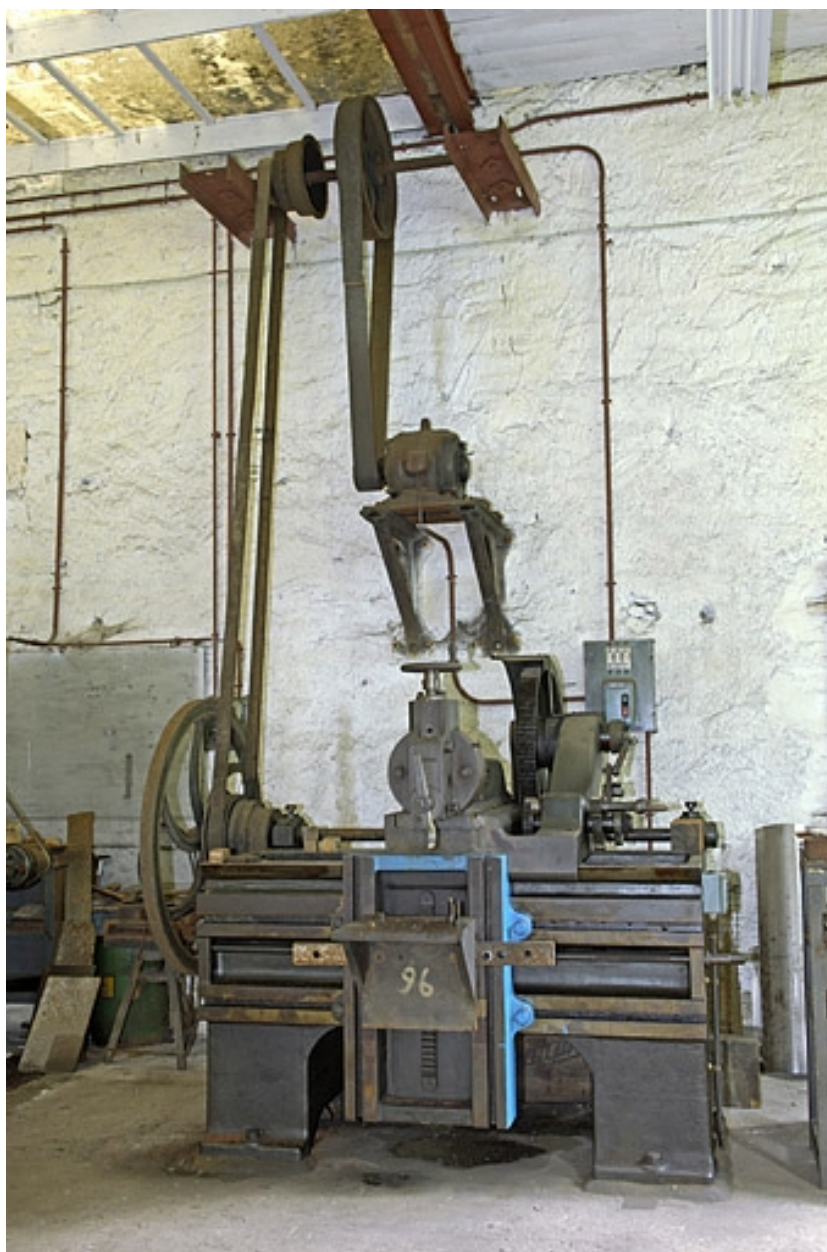
2e machine à usiner par outil de coupe (étou-limeur) : vue de face avec le moteur et sa transmission.
