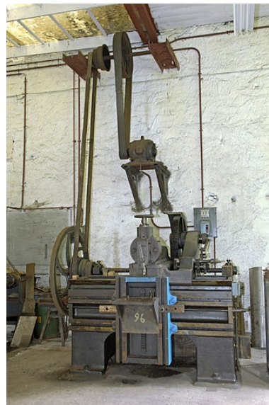
2e machine à usiner par outil de coupe (étau-limeur) : vue de face avec le moteur et sa transmission. Phot. Jérôme Mongreville IVR43_20057000215NUCA
