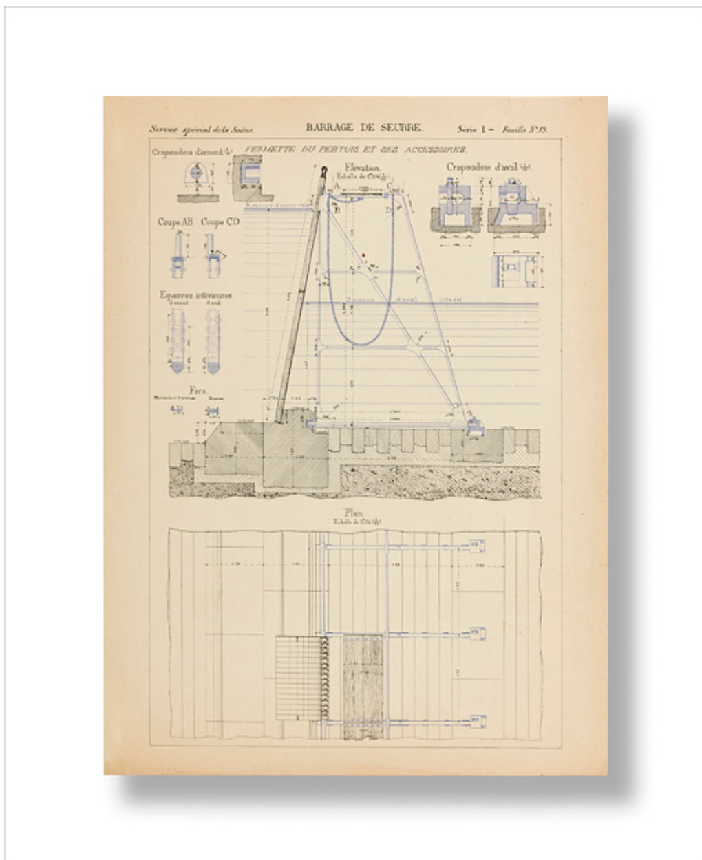
Barrage mobile de Seurre. Fermette du pertuis et ses accessoires. Plan, coupe et élévation.
