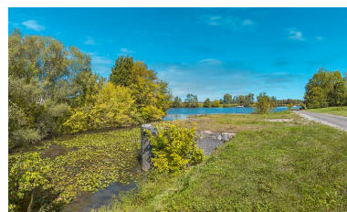
Les vestiges de la porte de garde de l'ancienne dérivation de Seurre. En arrière-plan, la Saône. Phot. Thierry Kuntz IVR26_20192100182NUC4A
