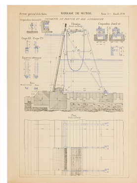
Barrage mobile de Seurre. Fermette du pertuis et ses accessoires. Plan, coupe et élévation. Phot. Thierry Kuntz IVR26_20172100136NUC4A
