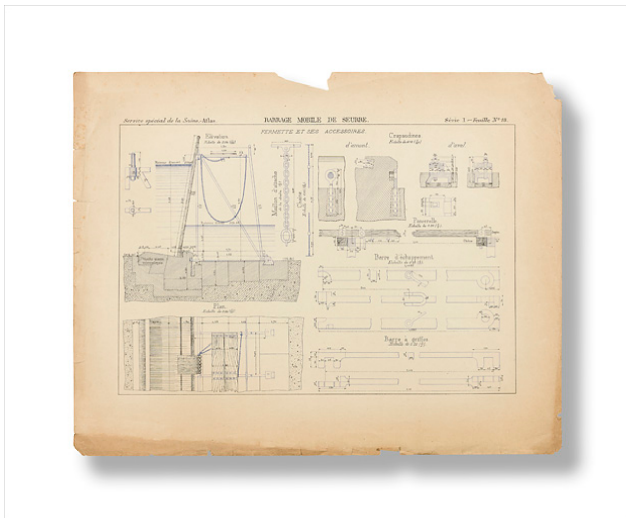
Barrage mobile de Seurre. Fermette et ses accessoires. Plan et élévation.
