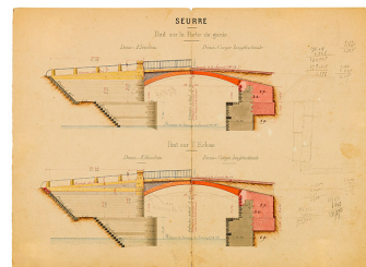
Elévations des ponts de Seurre. Pont sur la Porte de garde. Pont sur l'Ecluse. [Demi-élévation et demi-coupe longitudinale]. S.d.
