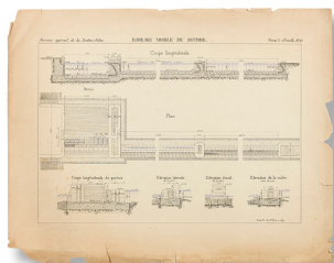
Barrage mobile de Seurre. Plan, coupe et élévation. Phot. Thierry Kuntz IVR26_20172100134NUC4A
