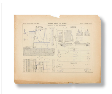
Barrage mobile de Seurre. Fermette et ses accessoires. Plan et élévation. Phot. Thierry Kuntz IVR26_20172100135NUC4A
