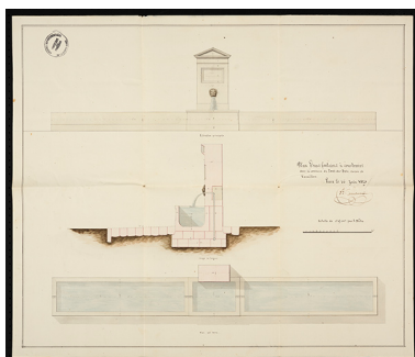
Plan d'une fontaine à construire (1829). Phot. Sonia Dourlot, Autr. A. Grandmougin IVR43_20167000018NUC4A
