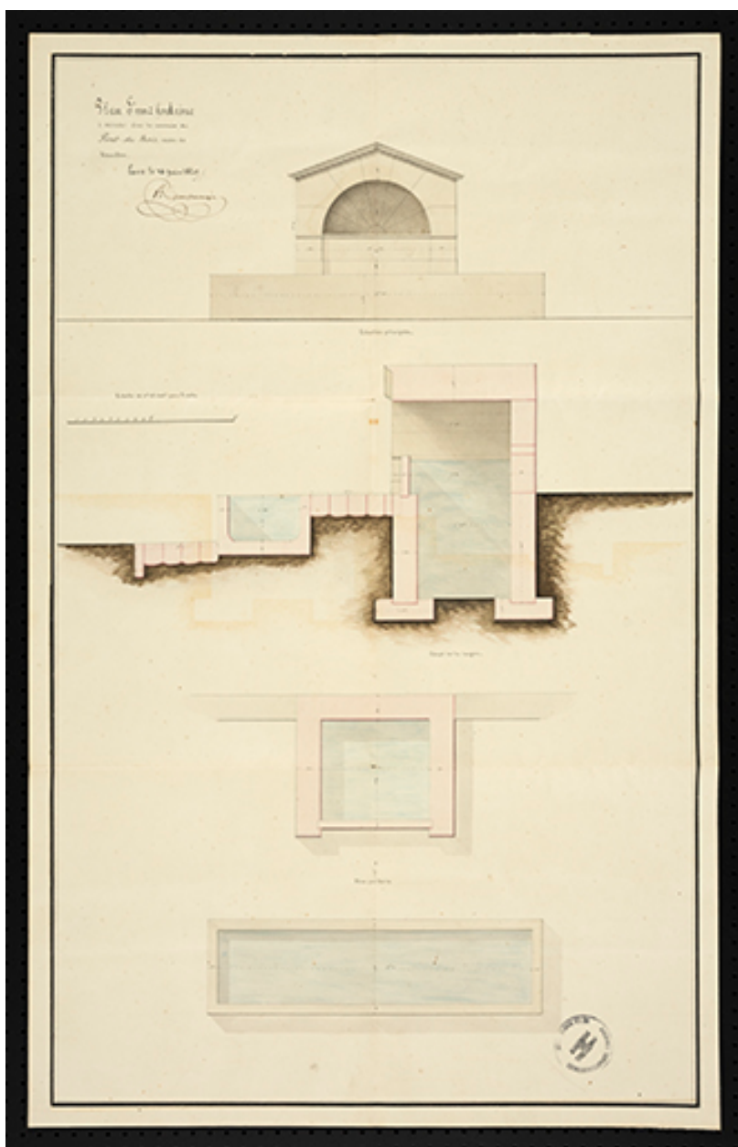
Plan d'une fontaine à construire, rue Saint-Nicolas (1829).
