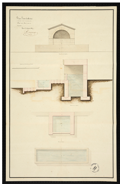
Plan d'une fontaine à construire, rue Saint-Nicolas (1829). Phot. Sonia Dourlot, Autr. A. Grandmougin IVR43_20167000017NUC4A
