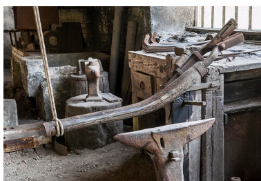
Cisaille de fabrication "maison". Reliée via une corde par une perche de noisetier fixée au plafond, elle est actionnée par le poids de l'ouvrier, assis en amazone sur le manche. Phot. Jérôme Mongreville IVR43_20152501544NUC4A
