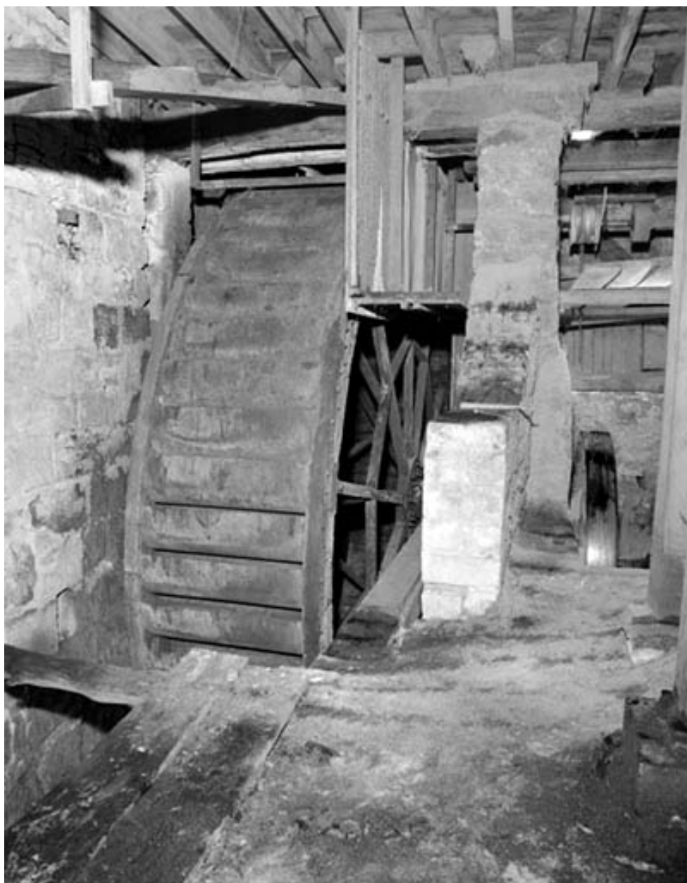
Bâtiment d'eau : la roue hydraulique.
