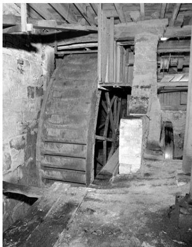
Bâtiment d'eau : la roue hydraulique. Phot. Yves Sancey IVR43_19973901236X
