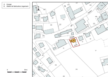
Plan-masse et de situation. Dess. Mathias Papigny IVR43_20162501517NUDA
