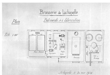
Brasserie de Lachapelle. Plan des bâtiments de fabrication. Phot. Jérôme Mongreville IVR43_20019000001V
