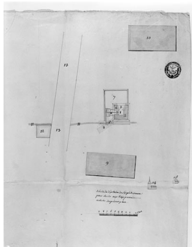
[Plan-masse du haut fourneau de Moutaine en 1797 d'après le] Plan d'un haut fourneau avec ses dépendances le tout couvert en thuilles [...]. Phot. Yves Sancey IVR43_19973901981V
