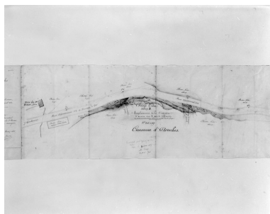
Plan des lieux à l'appui de la demande d'autorisation présentée par les sieurs Besson frères [...]. Phot. Yves Sancey IVR43_19973901985V
