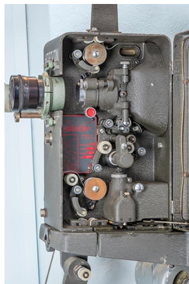
Mécanisme projecteur (système d'entraînement du film et objectif). Phot. Pierre-Marie Barbe-Richaud IVR26_20222100396NUC4A
