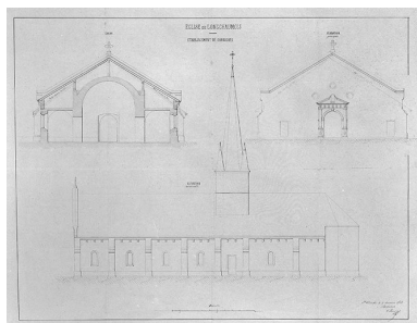
Eglise de Longchaumois : établissement de corniches, élévations, coupe, 1862. Phot. Jérôme Mongreville, Phot. Auguste Comoy IVR43_20013900332V
