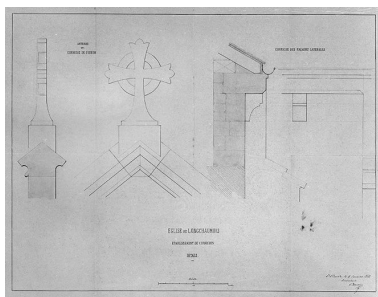
Eglise de Longchaumois : établissement de corniches, détails, 1862. Phot. Jérôme Mongreville, Phot. Auguste Comoy IVR43_20013900331V
