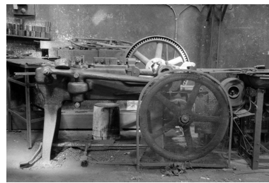
"Machine à rouler". Phot. Laurent Poupard IVR43_19893901249Z
