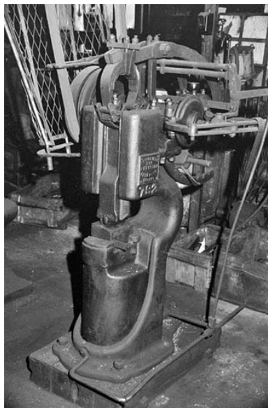
Marteau-pilon : détail. Plaque : Enköpings . Mek . Verkstad . Enköping . Patent . 792. Phot. Laurent Poupard IVR43_19893901247Z
