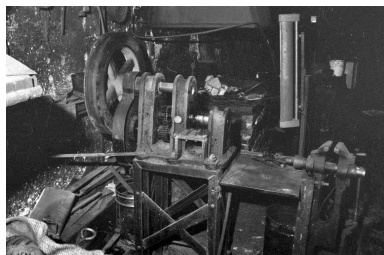
Laminoir. Phot. Laurent Poupard IVR43_19893901250Z
