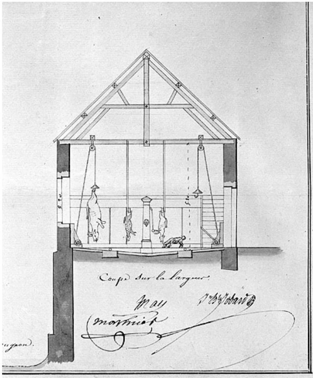
Plan et coupe du nouvel abattoir à construire [... Détail de la coupe]. 29 mai 1829.
