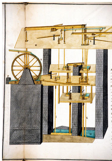
Machines Hydrauliques Qui Elèvent Les Eaux salées et douces du puit à Muire [détail du système d'élévation], 1756. Phot. Yves Sancey, Autr. Dorval IVR43_19943900218ZA
