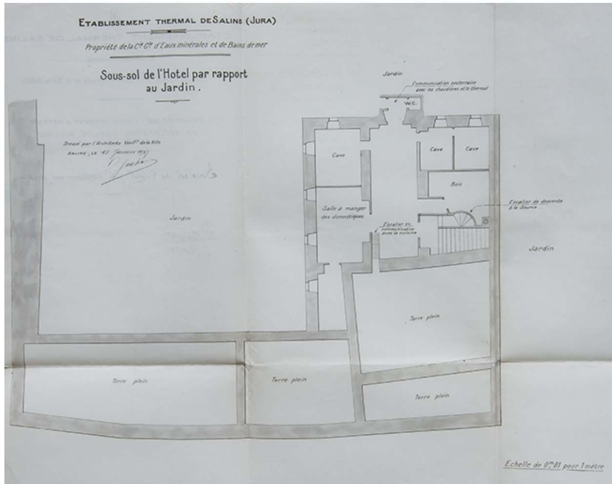
Plan du premier sous-sol (rez-de-jardin) du Grand Hôtel des Bains (1917).
