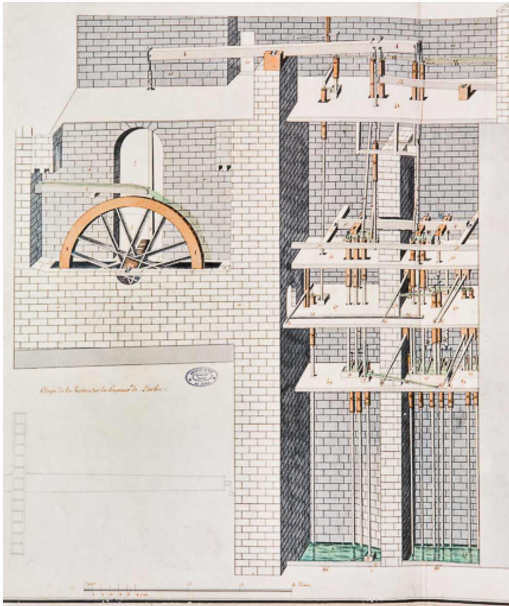
Machine hydraulique pour l'élévation des eaux salées et douces du Puits à muire [... : détail de la partie gauche], s.d. [18e siècle].
