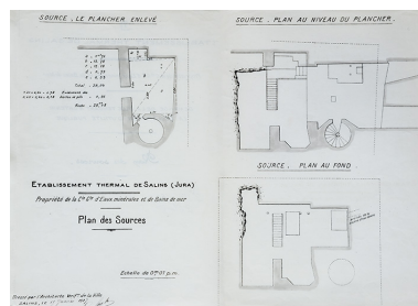
Plans du sous-sol du Grand Hôtel des Bains, figurant le puits à Muire (1917). Phot. Jérôme Mongreville IVR43_20223900084NUC4A
