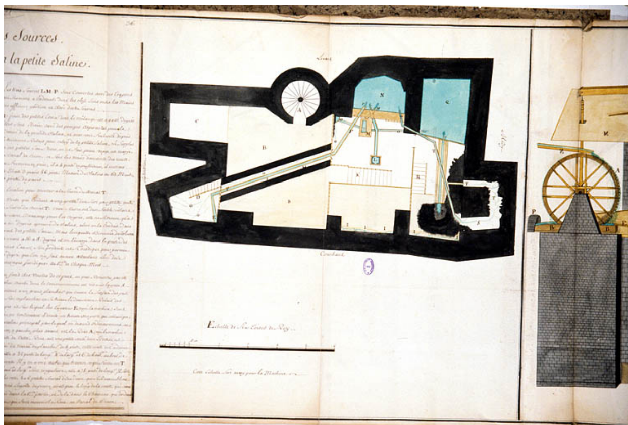
Machines Hydriques Qui Elèvent Les Eaux salées et douces du puits à Muire [plan du puits à muire], 1756.
