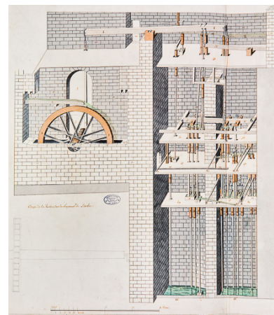
Machine hydraulique pour l'élévation des eaux salées et douces du Puits à muire [... : détail de la partie gauche], s.d. [18e siècle]. Phot. Yves Sancey IVR43_19943900526XA
