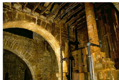
Parties supérieures du puits à Muire. Phot. Yves Sancey IVR43_19973902023ZA
