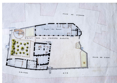
Plan de la saline en 1841. Phot. Jérôme Mongreville, Autr. Narcisse Perrard IVR43_20223900079NUC4A
