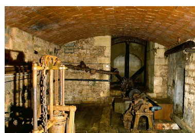
Plancher supérieur du puits à Muire. La roue hydraulique, visible au fond, actionnait une pompe située au fond du puits. Phot. Yves Sancey IVR43_19973902017ZA
