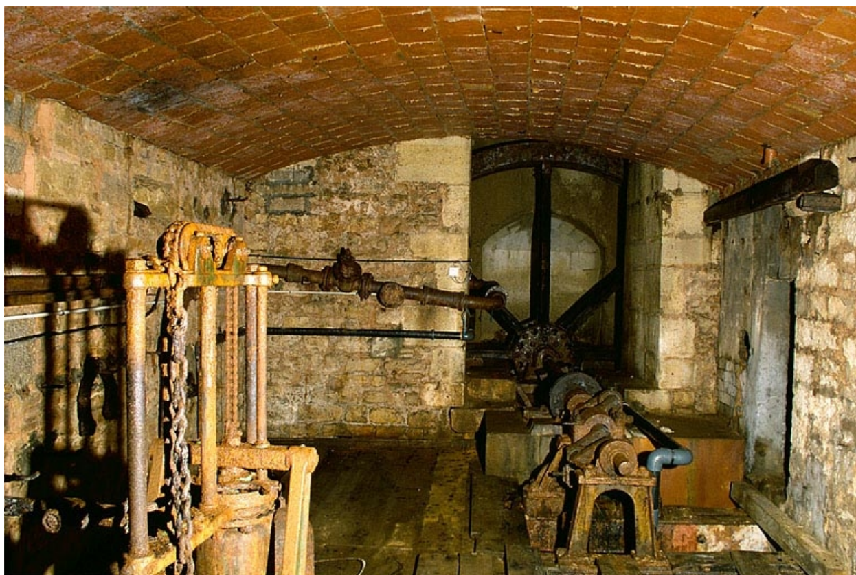
Plancher supérieur du puits à Muire. La roue hydraulique, visible au fond, actionnait une pompe située au fond du puits.
