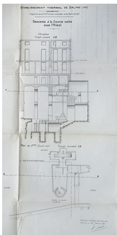
Coupes du sous-sol du Grand Hôtel des Bains, figurant le puits à Muire (1917). Phot. Jérôme Mongreville IVR43_20223900085NUC4A
