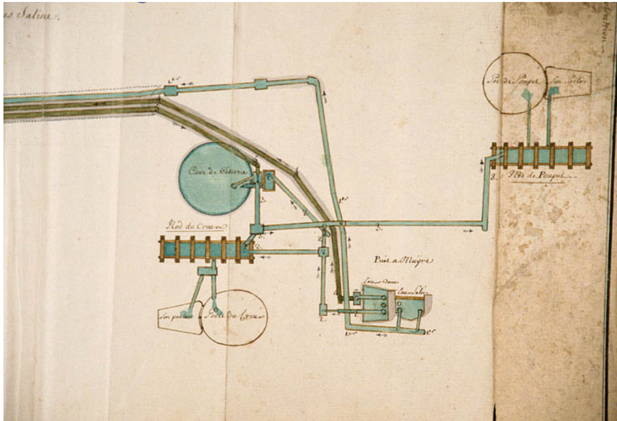
Plan des différents cours des eaux salées et douces des grande et petites salines de Salins [détail de la petite saline], 1756.
