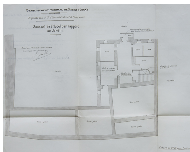
Plan du premier sous-sol (rez-de-jardin) du Grand Hôtel des Bains (1917). Phot. Jérôme Mongreville IVR43_20223900087NUC4A
