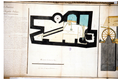
Machines Hydrauliques Qui Elèvent Les Eaux salées et douces du puit à Muire [plan du puits à muire], 1756. Phot. Yves Sancey, Autr. Dorval IVR43_19943900212ZA
