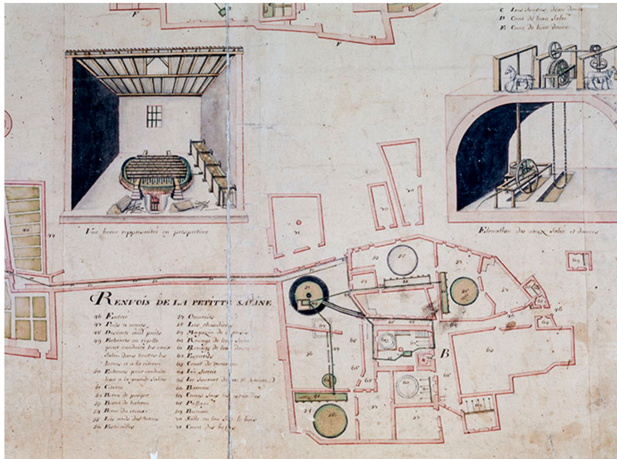
Plan géométral du Rets de chaussée de la grande et petite Saline de Salins [partie droite : la petite saline], 1718.
