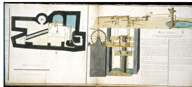
Machines Hydrauliques Qui Elèvent Les Eaux salées et douces du puit à Muire, 1756. Phot. Yves Sancey, Autr. Dorval IVR43_19943900209ZA
