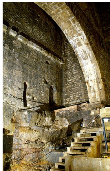
Mur sud du puits depuis le niveau inférieur. La principale source salée jaillit à gauche de l'escalier. Phot. Yves Sancey IVR43_19973902039ZA
