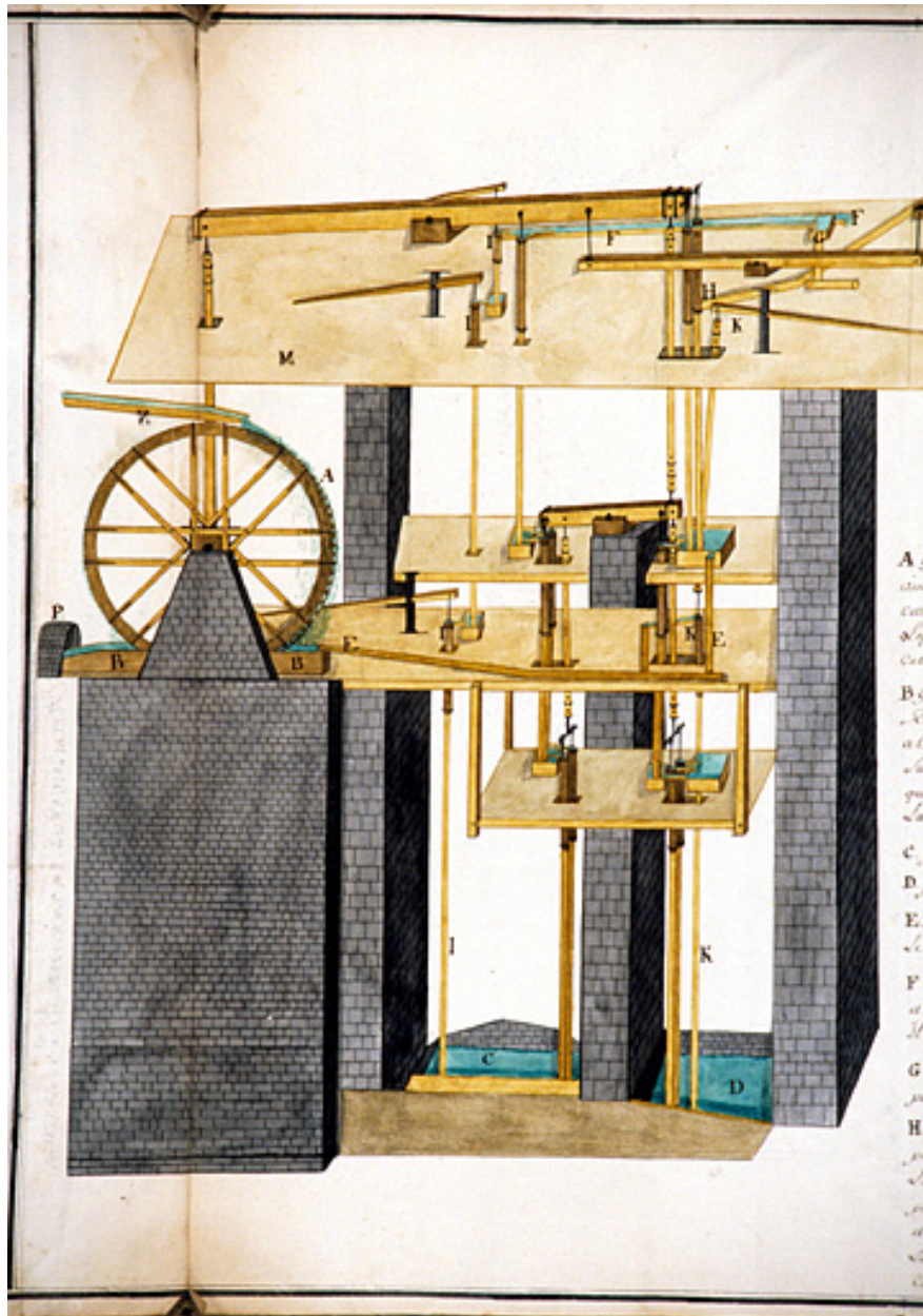
Machines Hydrauliques Qui Elèvent Les Eaux salées et douces du puits à Muire [détail du système d'élévation], 1756.
