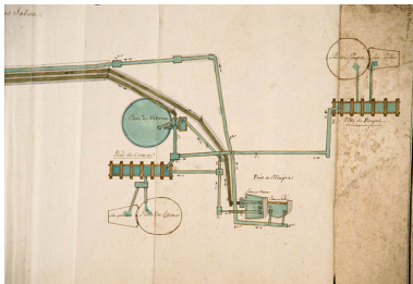
Plan des différents cours des eaux salées et douces des grande et petites salines de Salins [détail de la petite saline], 1756. Phot. Yves Sancey, Autr. Dorval IVR43_19943900184ZA
