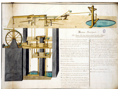
Machines Hydrauliques Qui Elèvent Les Eaux salées et douces du puit à Muire [partie droite], 1756. Phot. Yves Sancey, Autr. Dorval IVR43_19943900215ZA
