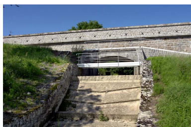
Déversoir de superficie du réservoir, prolongé par une chute d'eau en trois paliers et surmonté d'une passerelle. Phot. Alain Morelière IVR26_20072106043NUC2A
