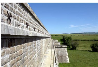
Le barrage et ses contreforts vu de l'extrémité est. Phot. Alain Morelière IVR26_20072106050NUC2A
