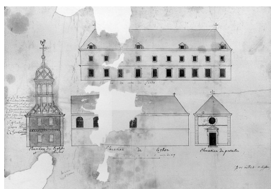
Elévation de l'église et du clocher [...], fin 17e siècle début 18e siècle. Phot. Yves Sancey, Autr. Claude- Antoine (architecte) Aillet IVR43_19842500004V
