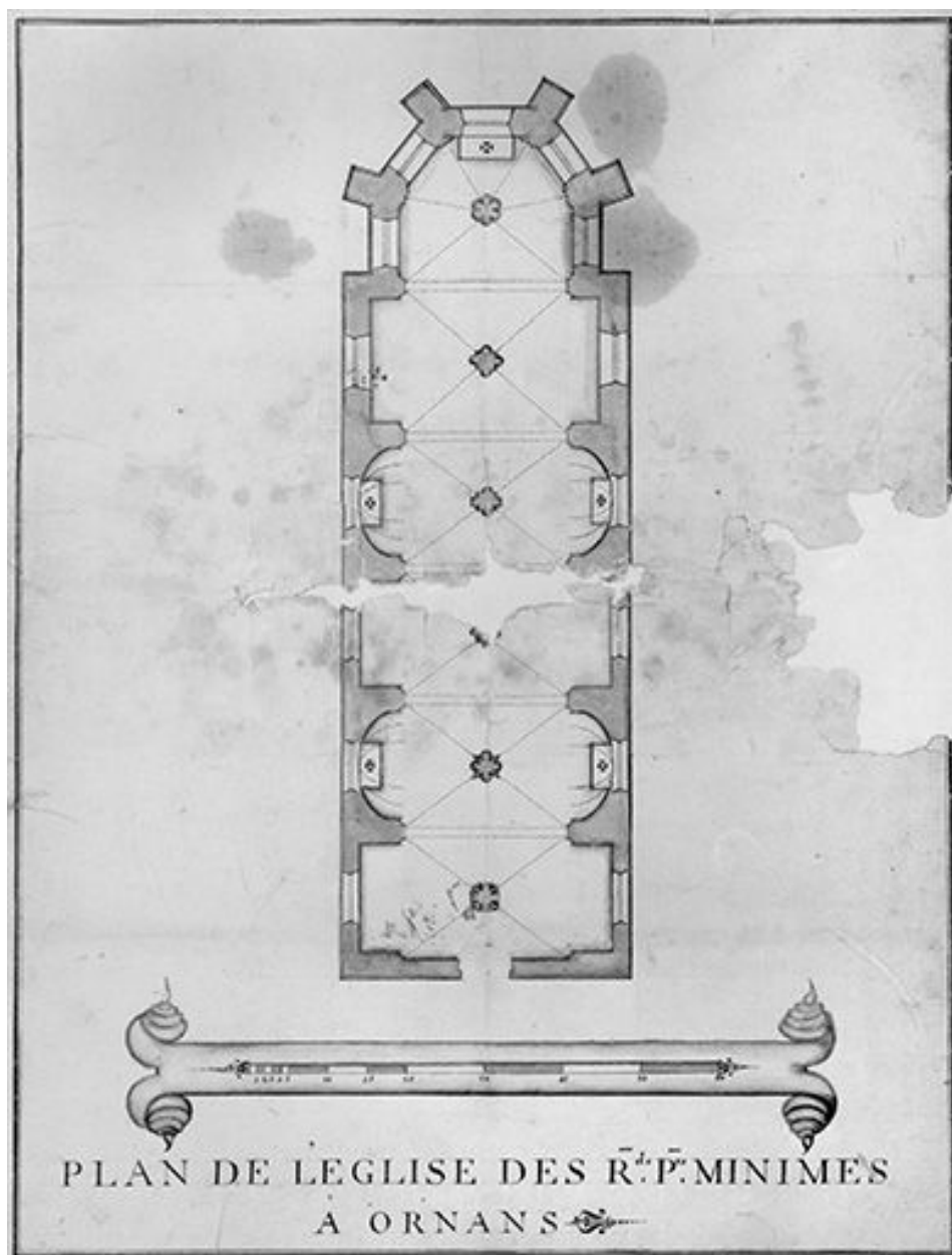
Plan de l'Eglise des Rds. Prs. Minimes à Ornans, 18e siècle.
