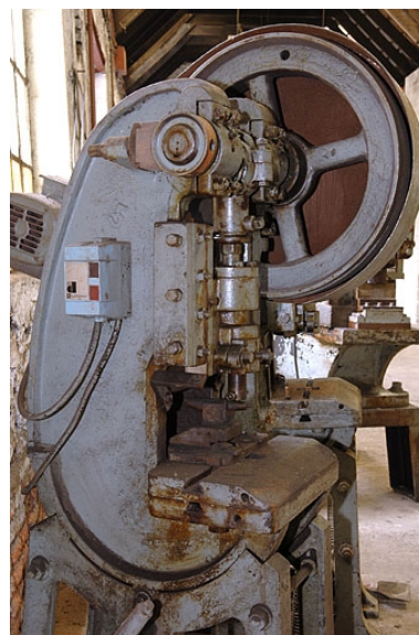
Vue de profil de la machine de gauche. Phot. Jérôme Mongreville IVR43_20057000076NUCA
