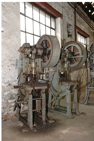
Vue de trois quarts gauche. Phot. Jérôme Mongreville IVR43_20057000088NUCA
