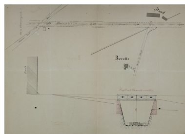
Plan à joindre à la demande de la société de tir de Champagnole [plan et élévation], 1882. Phot. Yves Sancey IVR43_20083900703NUC2A
