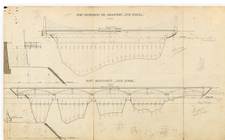
Pont suspendu de Chauvort et pont Me Boucicaut. 1897. Autr. Thevenard, Phot. Thierry Kuntz IVR26_20197100718NUC4A
