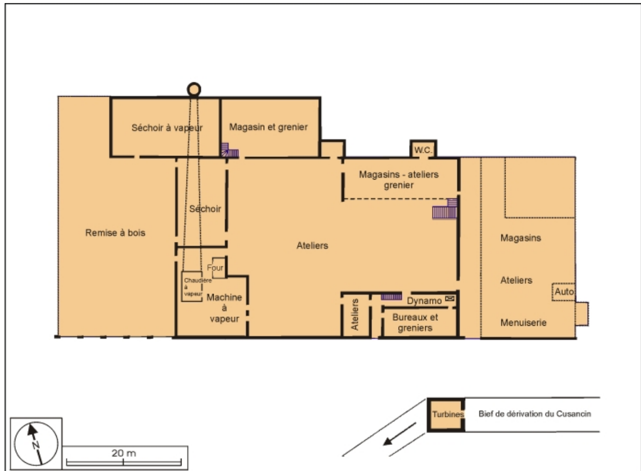
Plan-masse de l'usine (début du 20e siècle). D'après un plan de l'usine, mis au net par A. Céréza, échelle 1:600.
