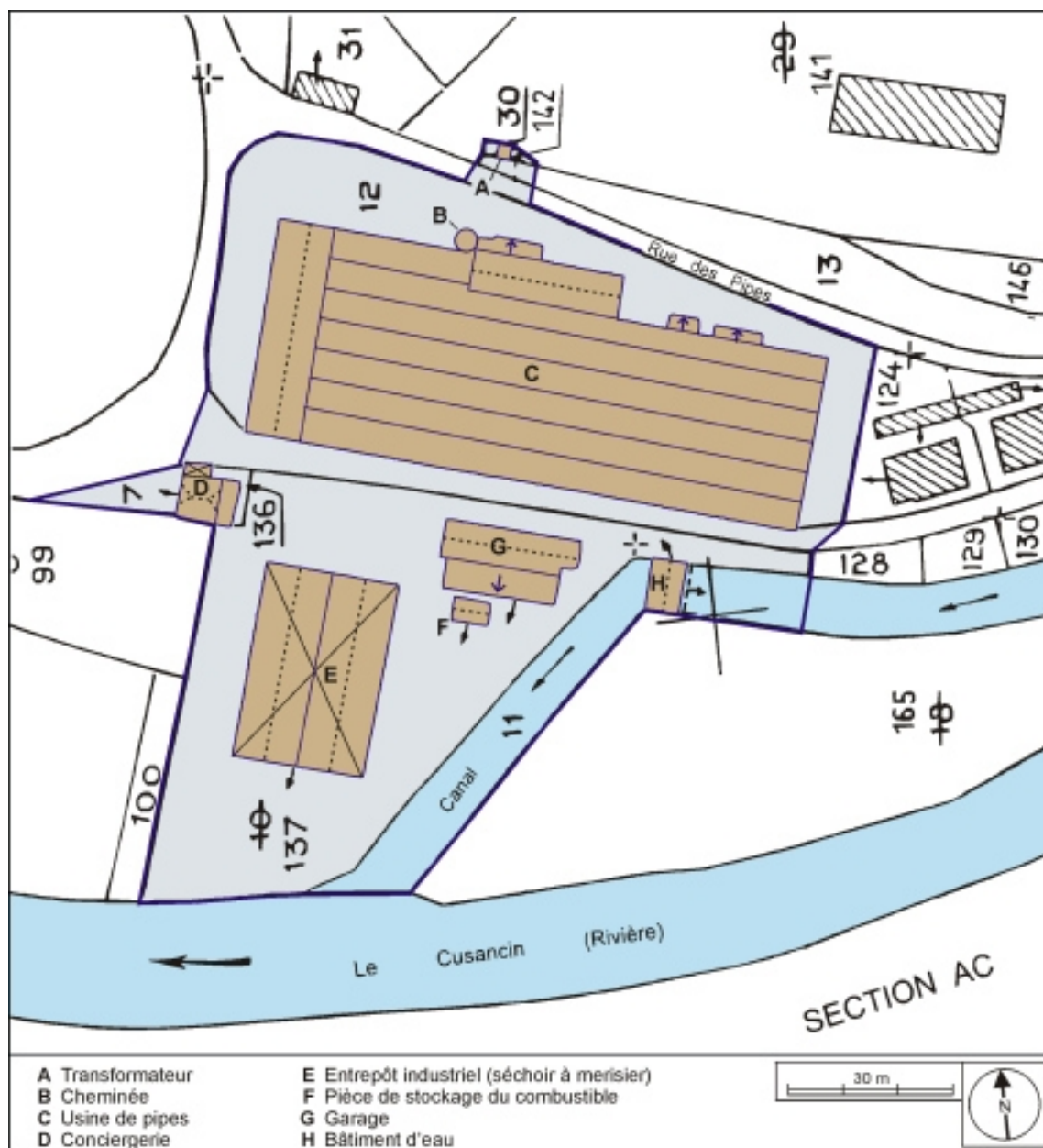
Plan-masse et de situation. Extrait du plan cadastral, 1982, section ZN, 1:2000 agrandi à 1:1000.
