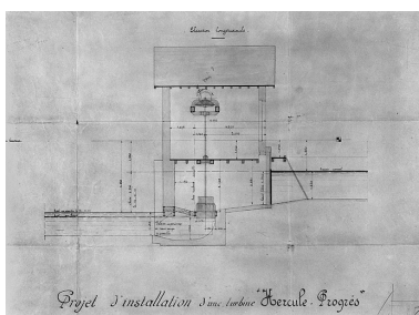
Projet d'installation d'une turbine Hercule-Progrès (Ets Singrün à Epinal), élévation longitudinale.
