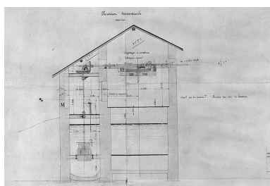
Projet d'installation d'une turbine Hercule-Progrès (Ets Singrün à Epinal), élévation transversale. Phot. Yves Sancey
