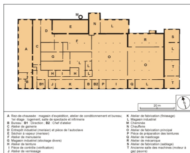
Plan-masse. D'après un plan de l'usine, mis à jour par A. Céréza, échelle 1:600. Dess. André Céréza IVR43_20022501343NUDA
