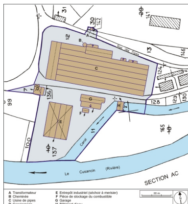
Plan-masse et de situation. Extrait du plan cadastral, 1982, section ZN, 1:2000 agrandi à 1:1000. Dess. André Céréza IVR43_20022501342NUDA
