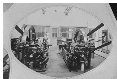
Salle des machines : moteurs à gaz pauvre. Phot. Yves Sancey
