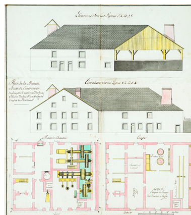
Plan de la maison basse de Consolation dans laquelle il existe deux moulins à blé, un moulin à scies, un feu de forge et un martinet [plans et élévations], s.d. [vers 1820]. Phot. Jérôme Mongreville IVR43_20152500575NUC4A
