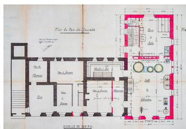
Projet de construction d'une fromagerie. Plan du rez-de-chaussée, 1919.
