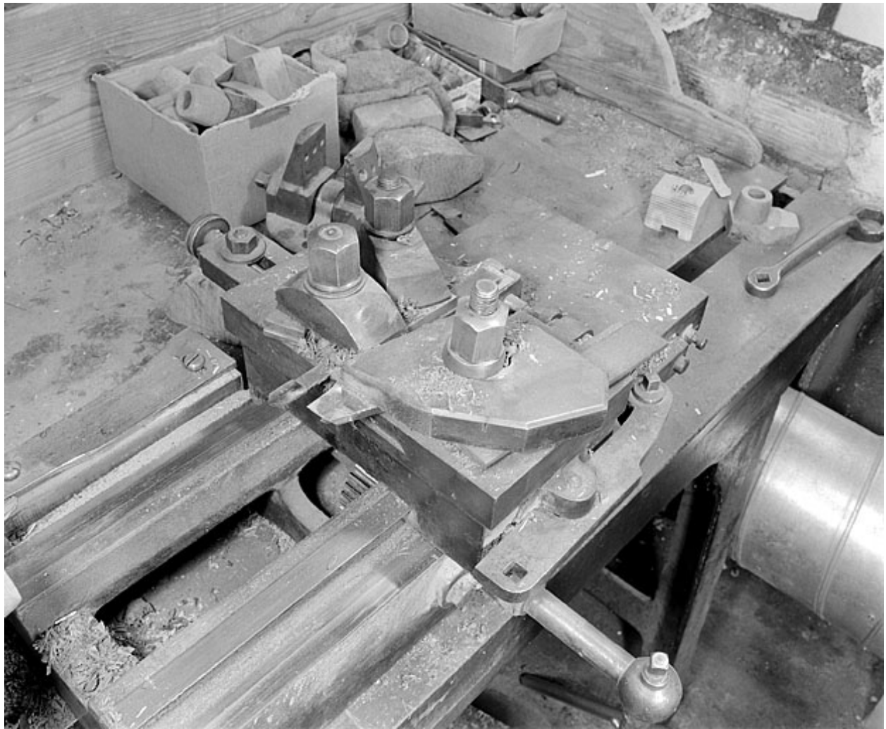
Chariot porte-outil (atelier de finissage).
