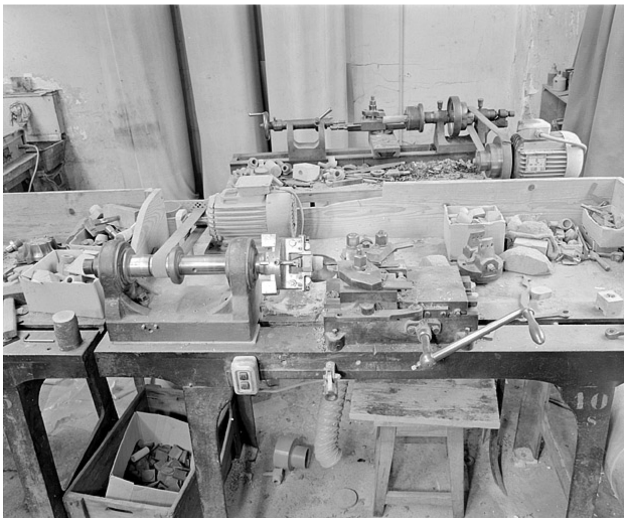
Vue d'ensemble du tour (atelier de finissage).
