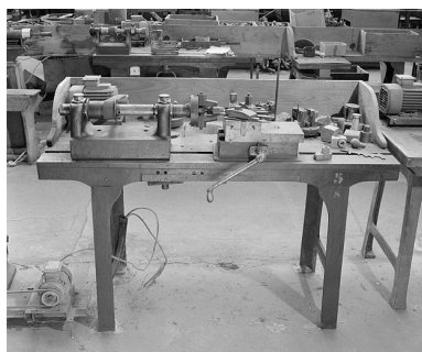
Vue d'ensemble du tour (atelier principal). Phot. Jérôme Mongreville IVR43_20022500633X
