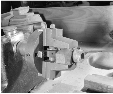
Mandrin "gueule de loup" (atelier principal). Phot. Jérôme Mongreville IVR43_20022500636X
