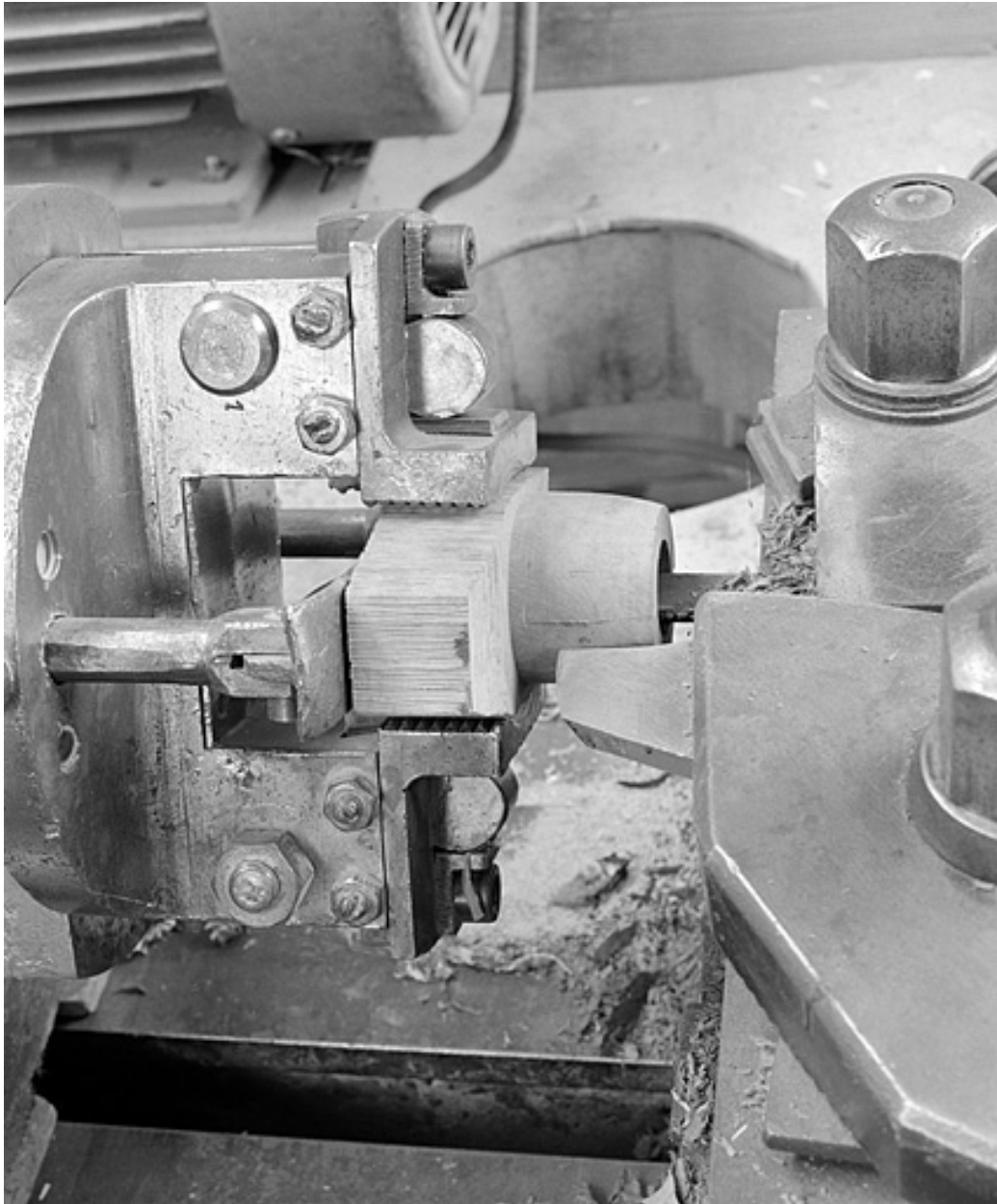
Détail du mandrin "gueule de loup" et du chariot porte-outil (atelier de finissage).
