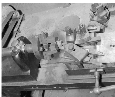
Mandrin "gueule de loup" et chariot porte-outil (atelier principal). Phot. Jérôme Mongreville IVR43_20022500635X
