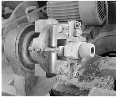
Mandrin "gueule de loup" (atelier de finissage). Phot. Jérôme Mongreville IVR43_20022500472X
