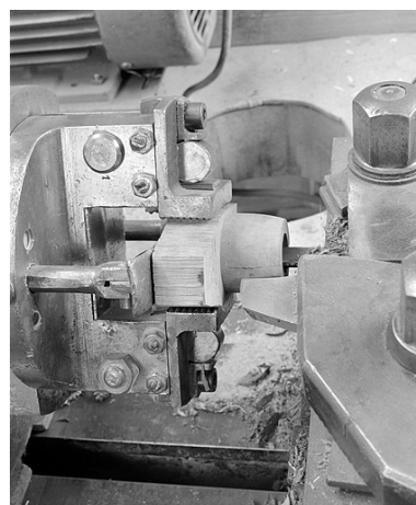
Détail du mandrin "gueule de loup" et du chariot porte- outil (atelier de finissage). Phot. Jérôme Mongreville IVR43_20022500473X
