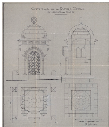
Projet d'Albert Salomon (1926), plan au sol, plan du couvrement, coupe et élévation. Autr. Albert Salomon, Phot. Jérôme Mongreville IVR43_20227000255NUC4A
