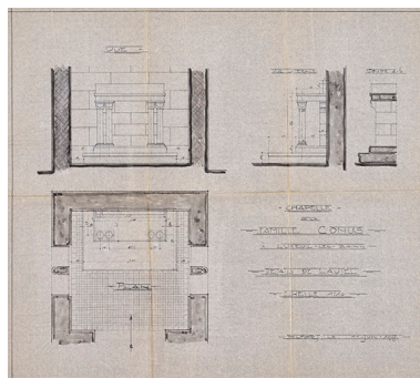
Projet d'Albert Salomon (1928), plan avec l'emplacement de l'autel. Autr. Albert Salomon, Phot. Jérôme Mongreville IVR43_20227000256NUC4A
