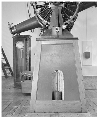
Pilier de la lunette, avec contrepoids visible. Phot. Jérôme Mongreville IVR43_20042500076X
