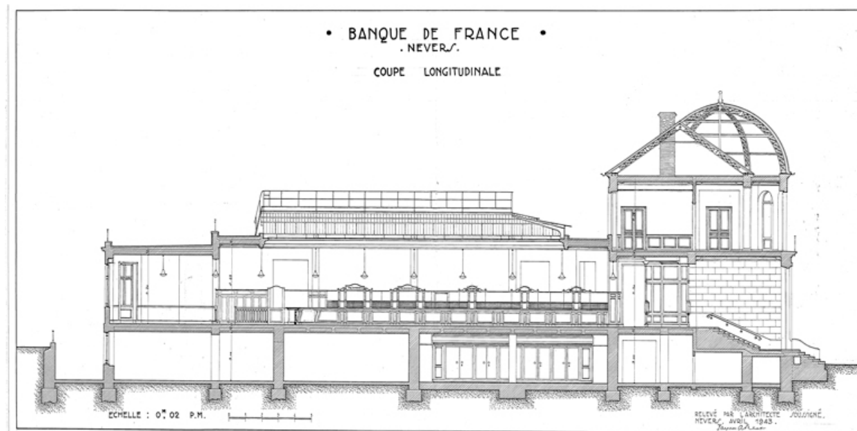
Coupe longitudinale (avril 1943).
