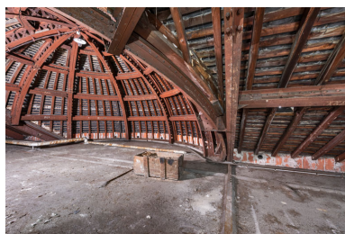
Charpente métallique. Phot. Pierre-Marie Barbe-Richaud IVR26_20235800041NUC4A
