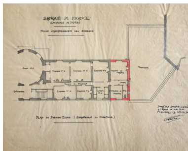
Plan du premier étage, projet d'extension (9 avril 1907). Autr. Auguste Palet, Phot. Fabien Dufoulon
