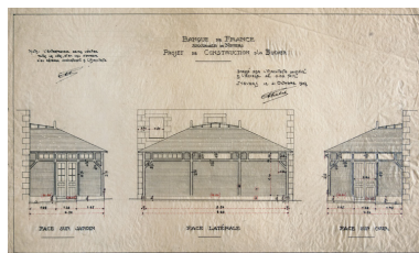
Élévations, projet de construction d'un bûcher (21 octobre 1907).
