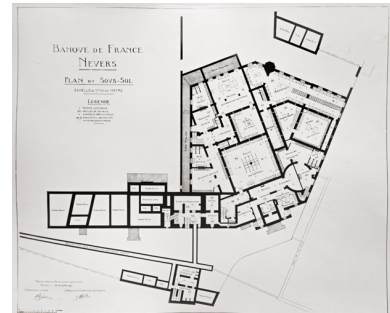
Plan du sous-sol (30 novembre 1927).
