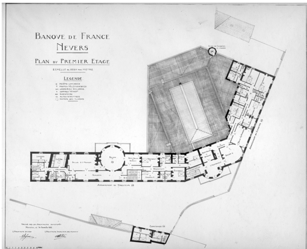
Plan du premier étage (30 novembre 1927).
