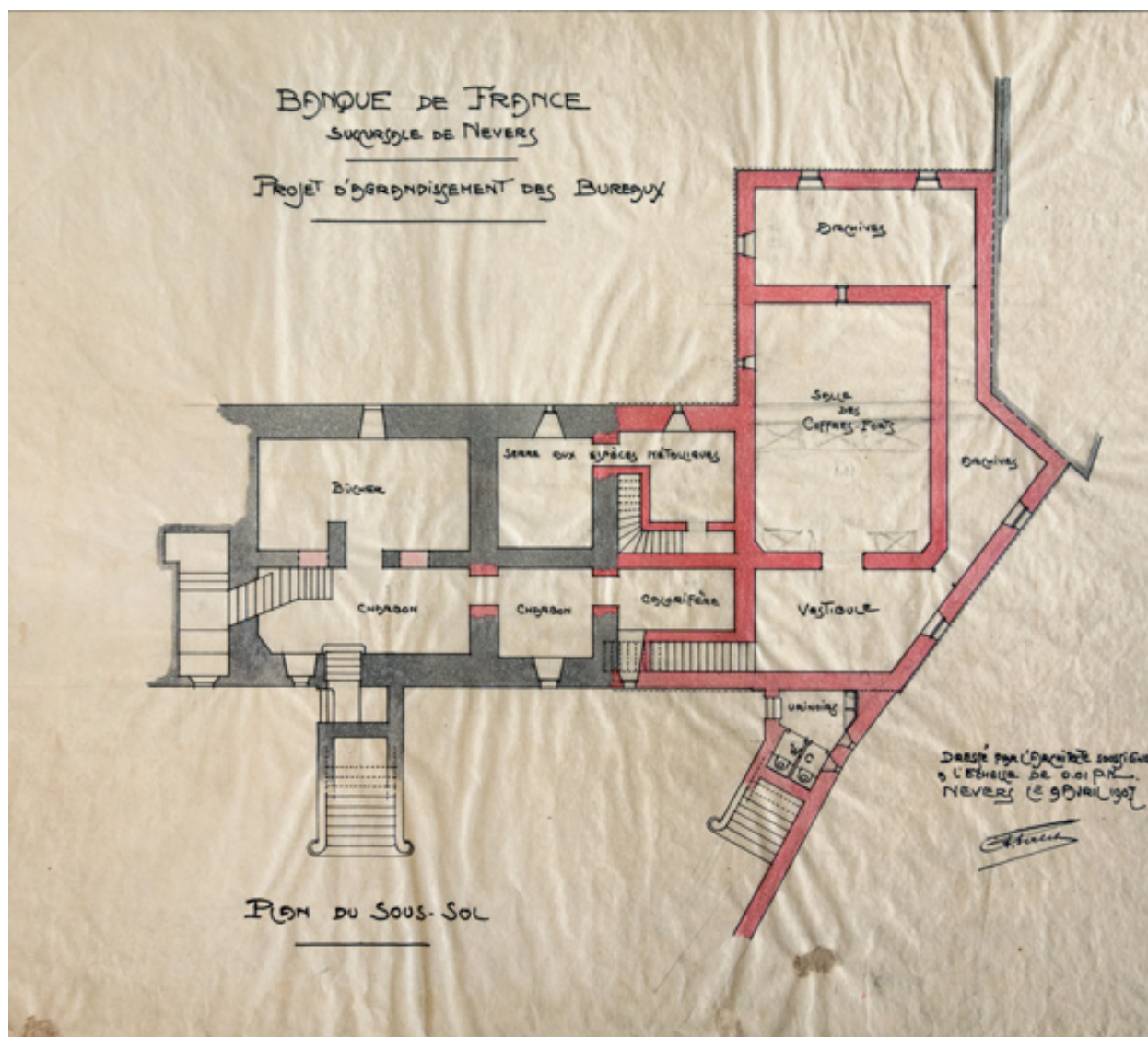
Plan du sous-sol, projet d'extension (9 avril 1907).
