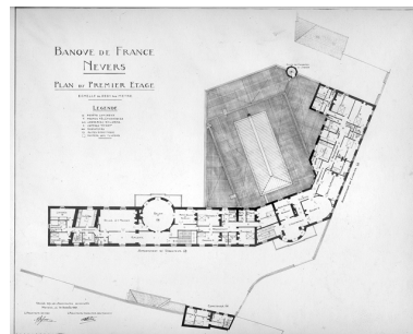
Plan du premier étage (30 novembre 1927).
