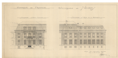
Façade sur la rue, projet d'extension (15 janvier 1924).
