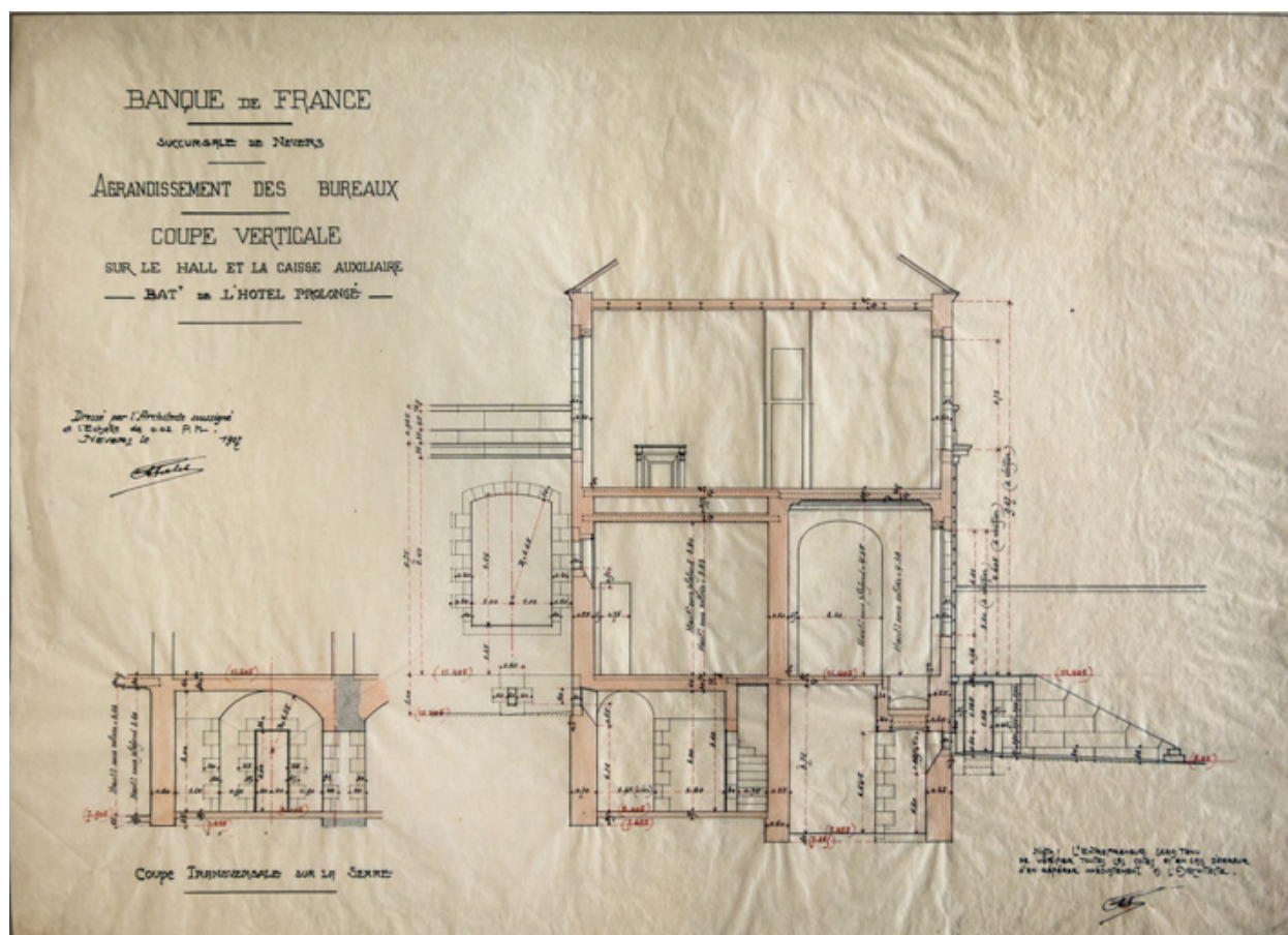
Coupe sur le hall et la caisse auxiliaire, projet d'extension (1907).
