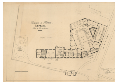
Plan du rez-de-chaussée, projet d'extension (10 juin 1921).
