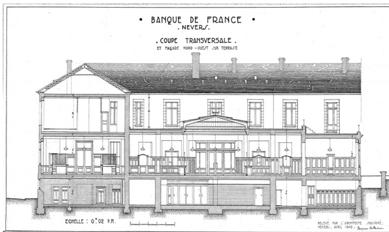
Coupe transversale (avril 1943).
