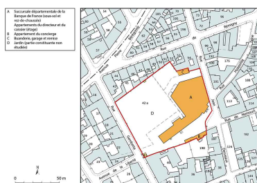
Plan-masse et de situation, extrait du plan cadastral (2023). Dess. Aline Thomas
