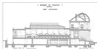
Coupe longitudinale (avril 1943).
