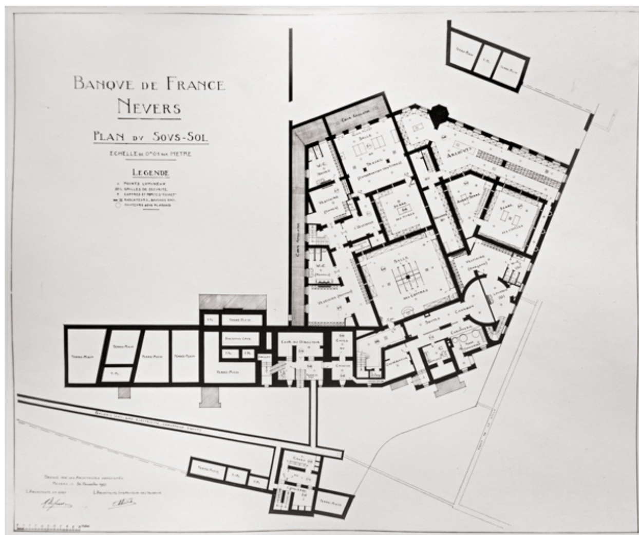
Plan du sous-sol (30 novembre 1927).
