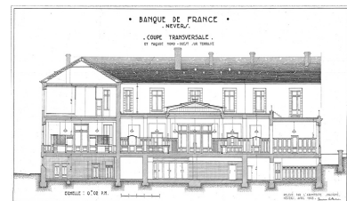
Coupe transversale (avril 1943).
