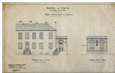
Façade sur la cour, projet d'extension (9 avril 1907). Autr. Auguste Palet, Phot. Fabien Dufoulon IVR26_20235800113NUC2A
