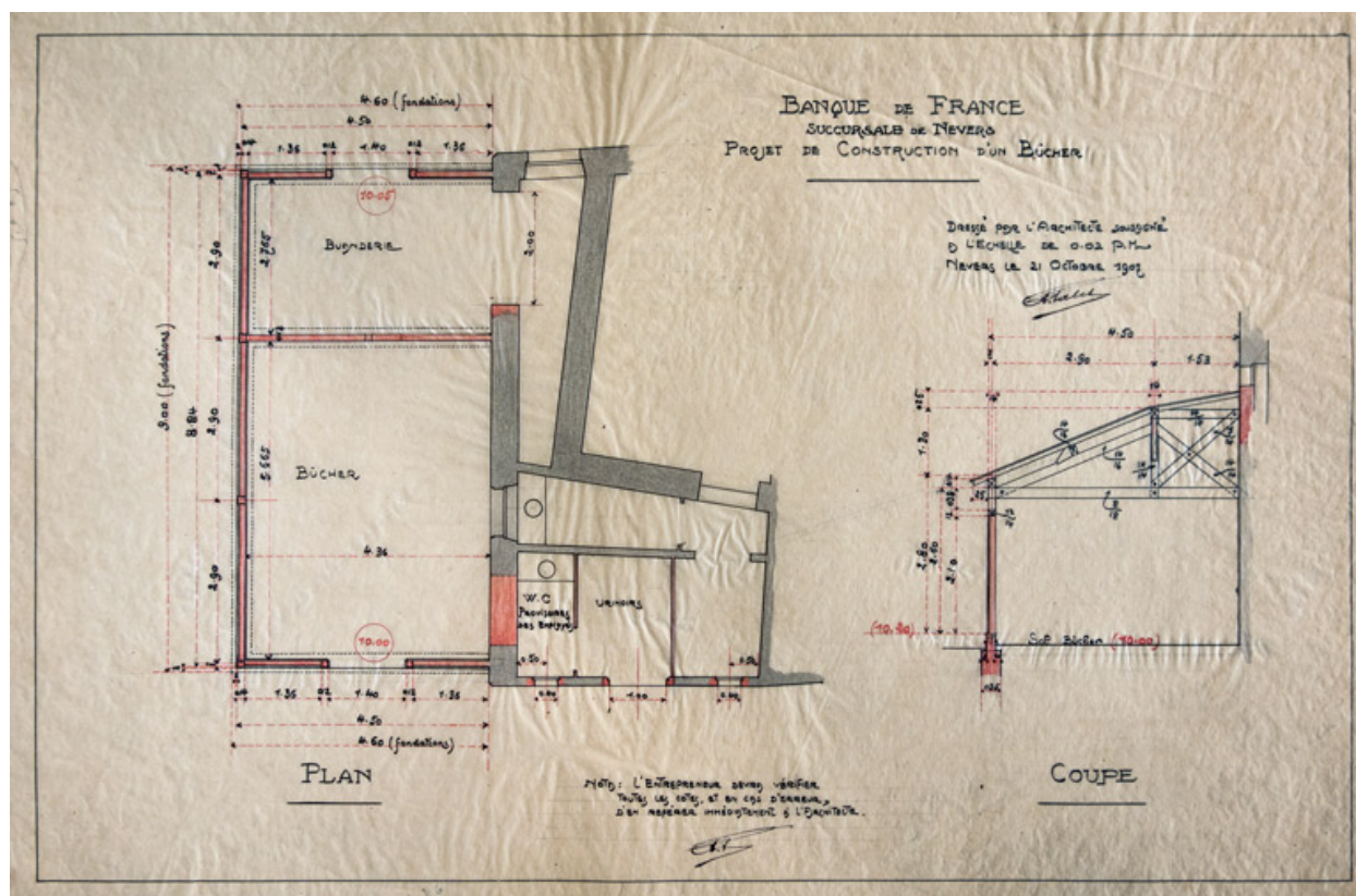
Plan et coupe, projet de construction d'un bûcher (21 octobre 1907).
