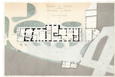
Plan du rez-de-chaussée (1895). Autr. J. Boutée IVR26_20235800134NUC4A
