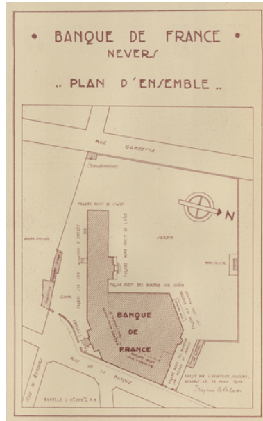
Plan-masse et de situation (1943).
