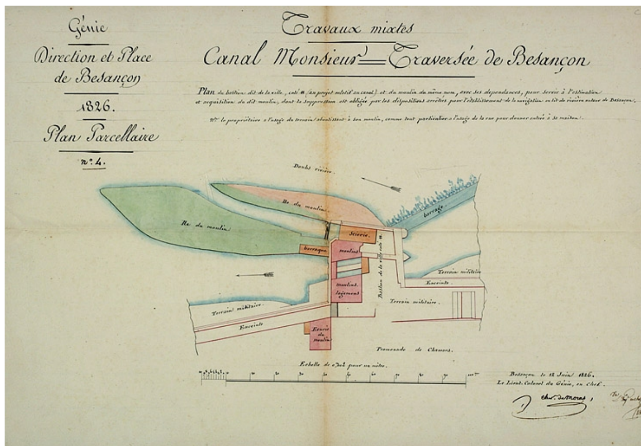
Plan du bastion dit de la Ville, cotti 11 (au projet relatif au canal), et du moulin du même nom [...], 1826.
