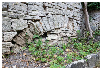
Détail de la maçonnerie d'une voûte. Phot. Jérôme Mongreville IVR43_20177000836NUC4A
