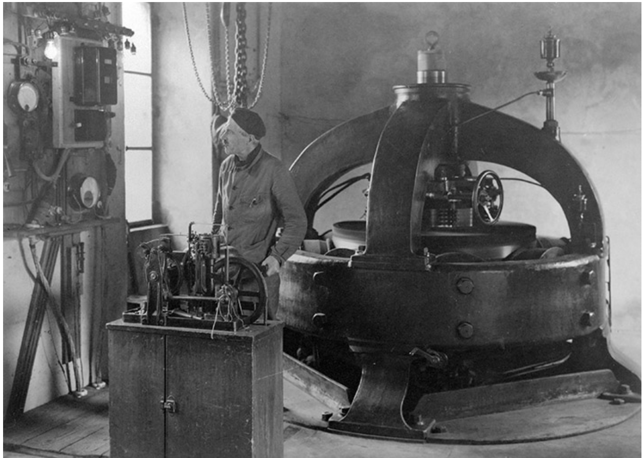
[Centrale hydroélectrique de la Roche] Dynamo de 110 Kw datant de 1891, 1950-1951.
