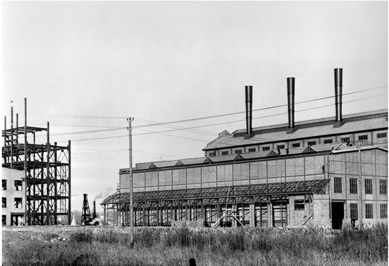
[Tavaux et Abergement-la-Ronce] Générateurs de vapeur et d'électricité de l'usine Solvay en construction, 23 janvier 1930.
