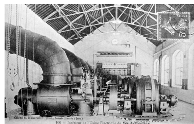
Intérieur de l'Usine Electrique du Saut-Mortier, [limite 19e siècle 20e siècle, entre 1898 et 1911]. Phot. Yves Sancey, Autr. E. (photographe) NEPASUTILISERMandrillon IVR43_19883900434X
