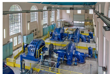
Centrale hydroélectrique du Refrain, Charquemont : intérieur. Phot. Yves Sancey IVR43_20122502140NUC2A
