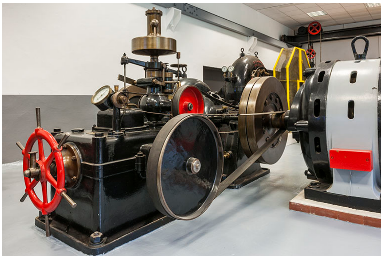
Centrale du Fourpéret, Labergement-Sainte-Marie : régulateur SACM et son alternateur.
