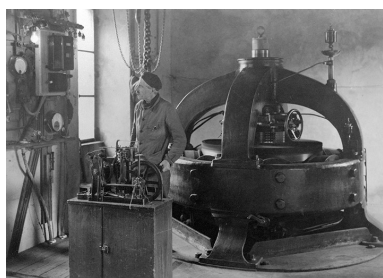
[Centrale hydroélectrique de la Roche] Dynamo de 110 Kw datant de 1891, 1950-1951. Phot. Yves Sancey, Autr. R. Ponget IVR43_19883900722V
