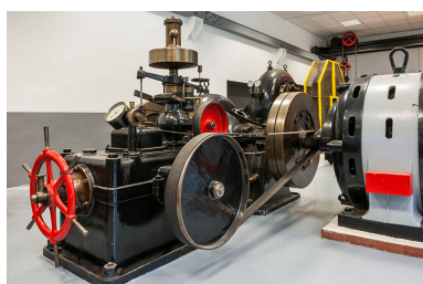
Scierie Renaud puis centrale hydroélectrique Huot-Marchand, Battenans-Varin. Phot. Yves Sancey IVR43_20132501153NUC2A
