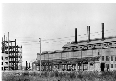
[Tavaux et Abergement-la-Ronce] Générateurs de vapeur et d'électricité de l'usine Solvay en construction, 23 janvier 1930. Phot. Jérôme Mongreville, Phot. Charnotet IVR43_19903900039X
