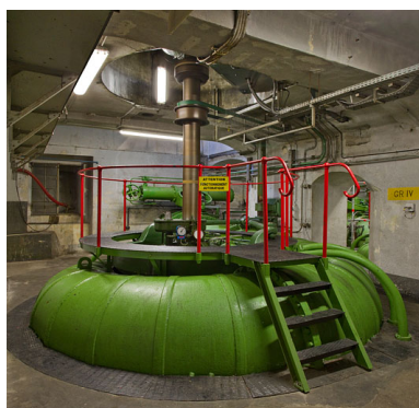
Centrale hydroélectrique de Liebwillers : bâche de turbine à l'étage de soubassement.
