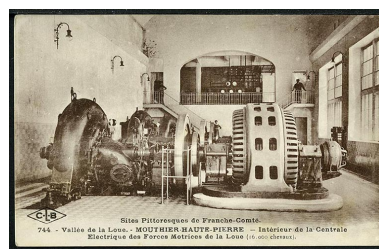
Vallée de la Loue - Mouthier-Haute- Pierre. Intérieur de la Centrale Electrique des Forces Motrices de la Loue, [début 20e siècle]. IVR43_20182500296NUC2A
