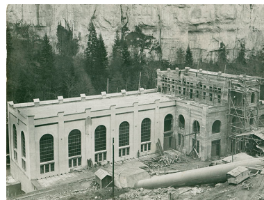
[Centrale du Refrain en construction, Charquemont], [1908 ou 1909]. Autr. auteur inconnu IVR43_20172500015NUC4A
