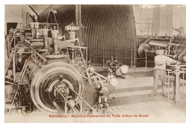
Ronchamp. - Machine d'Extraction du Puits Arthur de Buyer, [avant 1923]. Phot. Jérôme Mongreville IVR43_20057000633NUCA
