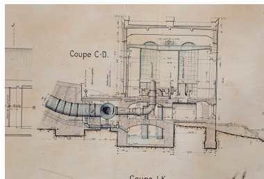
Forces motrices du Refrain. Usine [détail : coupe transversale], 1908. Phot. Yves Sancey, Autr. Société des Forces motrices de l'Est IVR43_20122502174NUC2A
