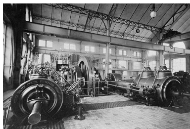
[Centrale électrique, Besançon (23 avenue Arthur Gaulard) : machine à vapeur et dynamo], [début 20e siècle]. Phot. Yves Sancey IVR43_19882500241V
