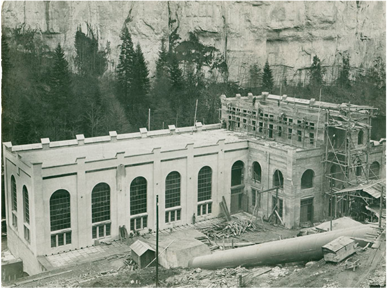
[Centrale du Refrain en construction, Charquemont], [1908 ou 1909].
