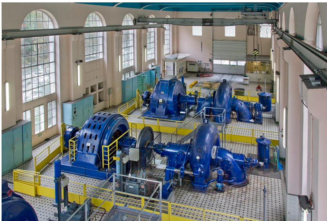
Centrale hydroélectrique du Refrain, Charquemont : intérieur.
