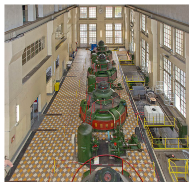
Centrale hydroélectrique de Liebwillers : intérieur.
