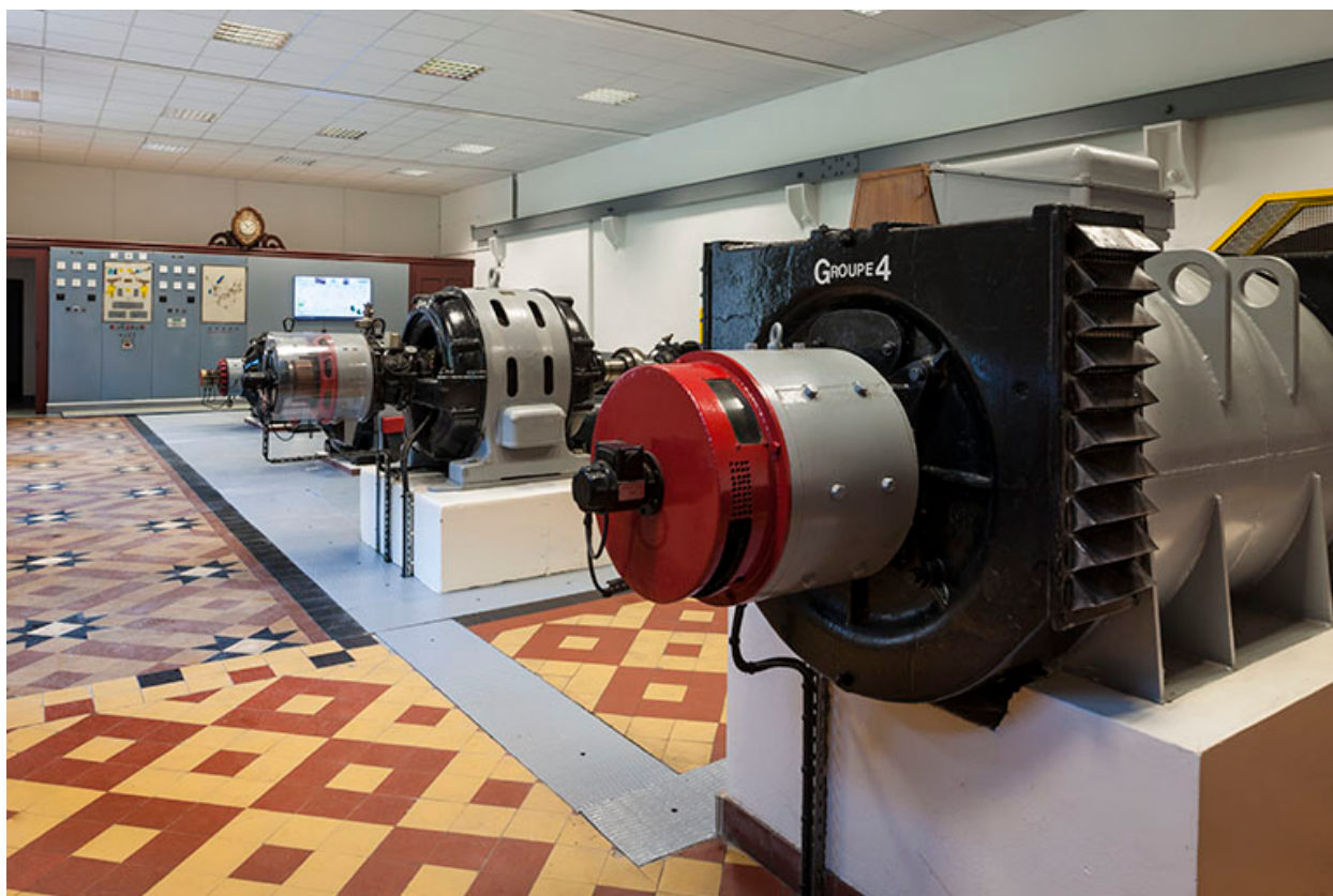
Centrale du Fourpéret, Labergement-Sainte-Marie : intérieur.
