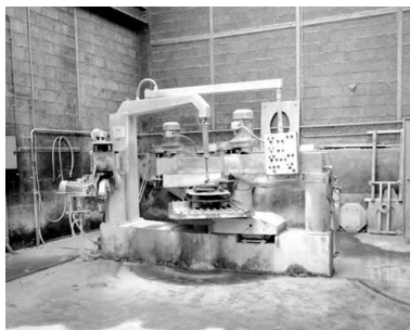
Machine prête à fonctionner. Phot. Yves Sancey IVR43_19933900356X
