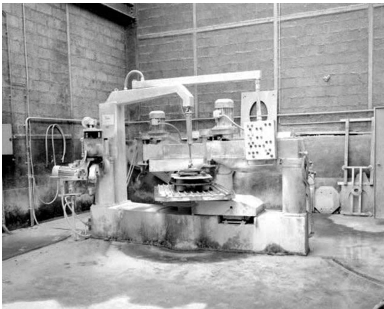
Machine prête à fonctionner.
