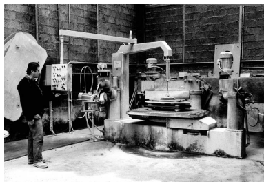
Vue d'ensemble, avec ouvrier. Phot. Yves Sancey IVR43_19933900491ZA
